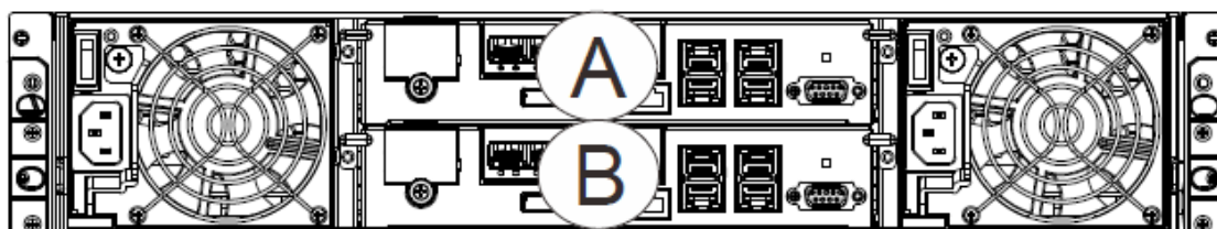
图 1- 2.GS5324M 后视图
