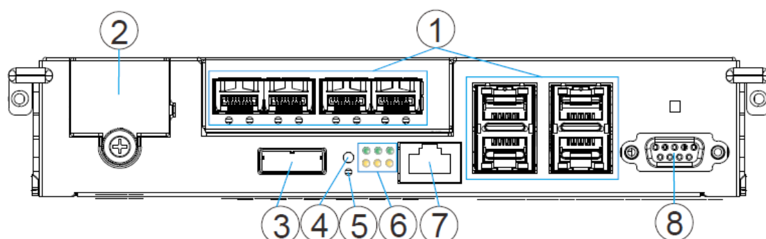
图 1- 6.控制器组成
