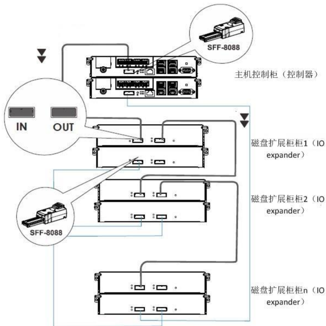
图 1- 7.GS5324M 扩展柜连接示意图
