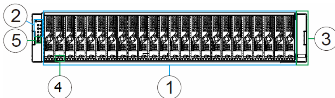
图 1- 3.GS5324M 前视图组件分布
