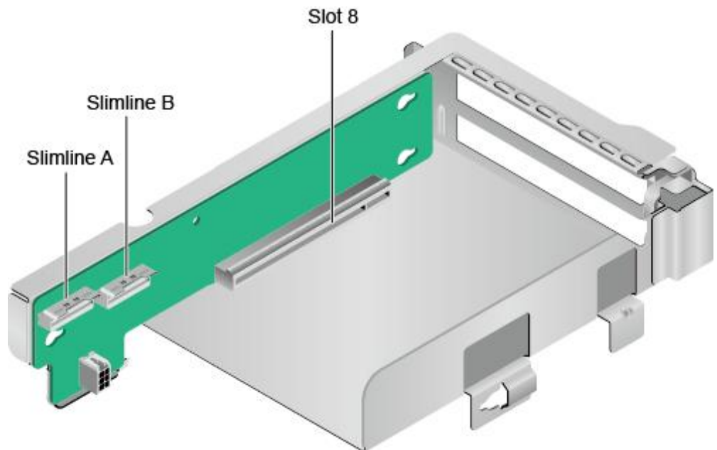
图 5-34 1x16 Riser 卡 7
