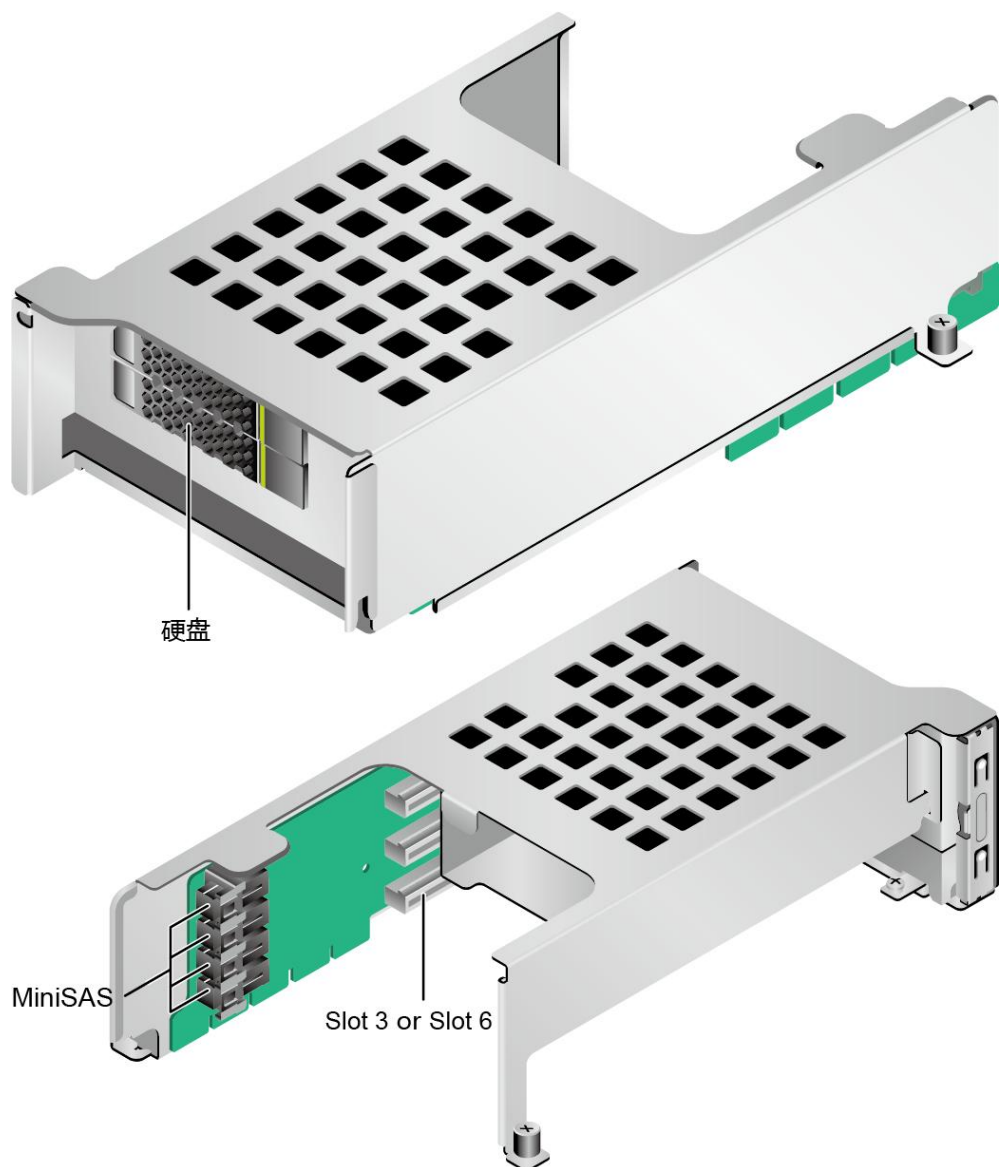
图 5-32 SAS Riser 卡 5
