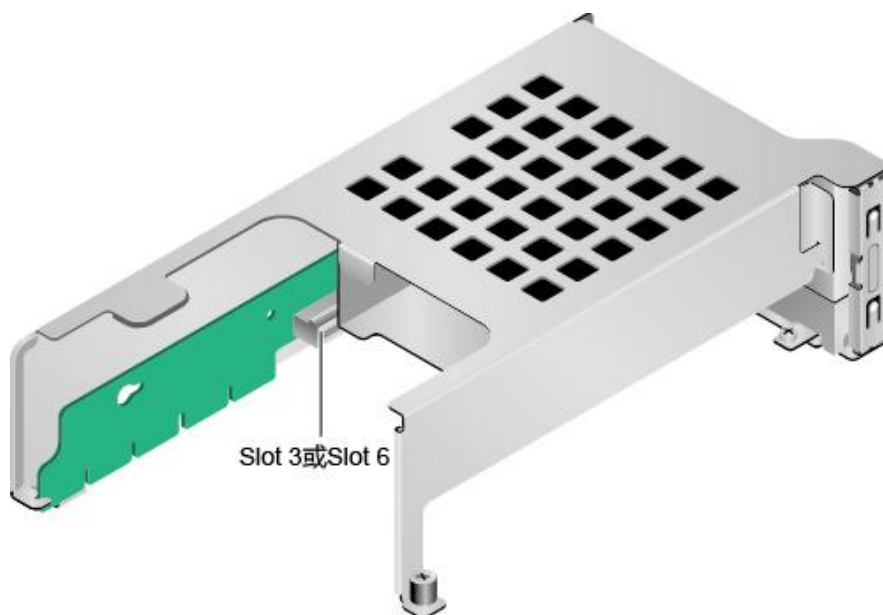
图 5-31 1x16 Riser 卡 4
