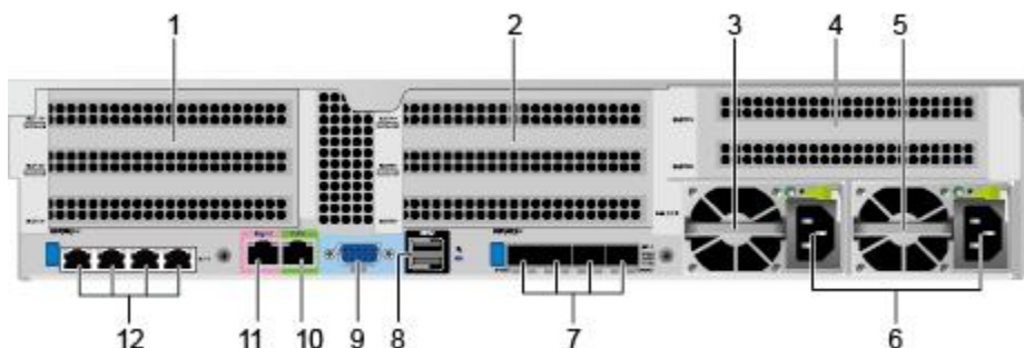
图 5-13 后面板组件
