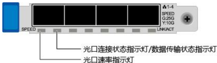
图 5-16 TM280 (4x25GE 光口)
