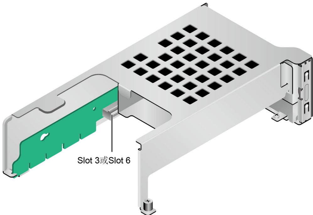
图 4-11 Riser 卡 3 (1x16)
