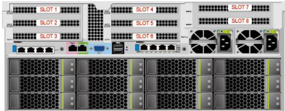
图 4-14 PCIe 插槽
