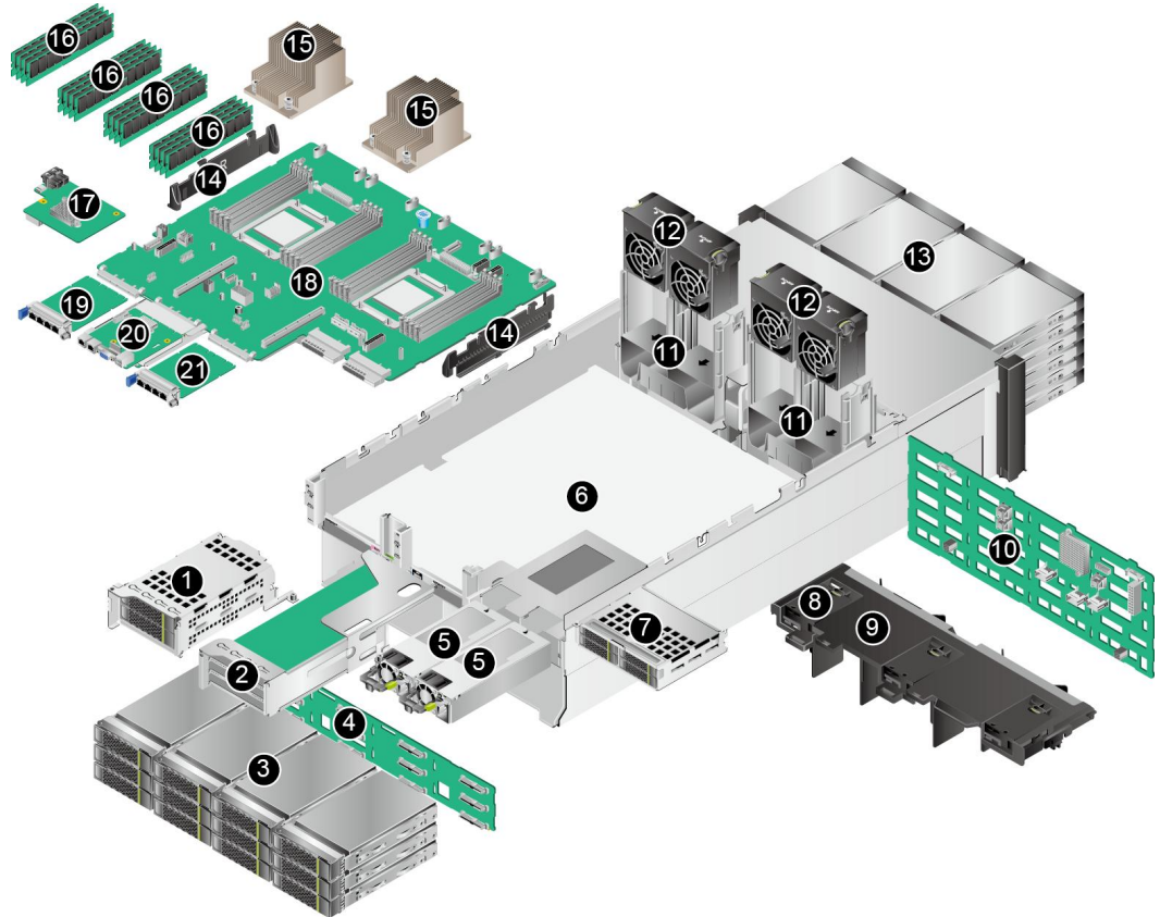
图 4-15 部件
