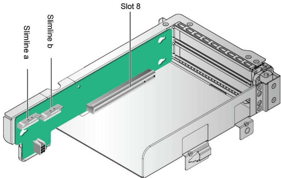
图 4-13 Riser 卡 6 (1x16)
