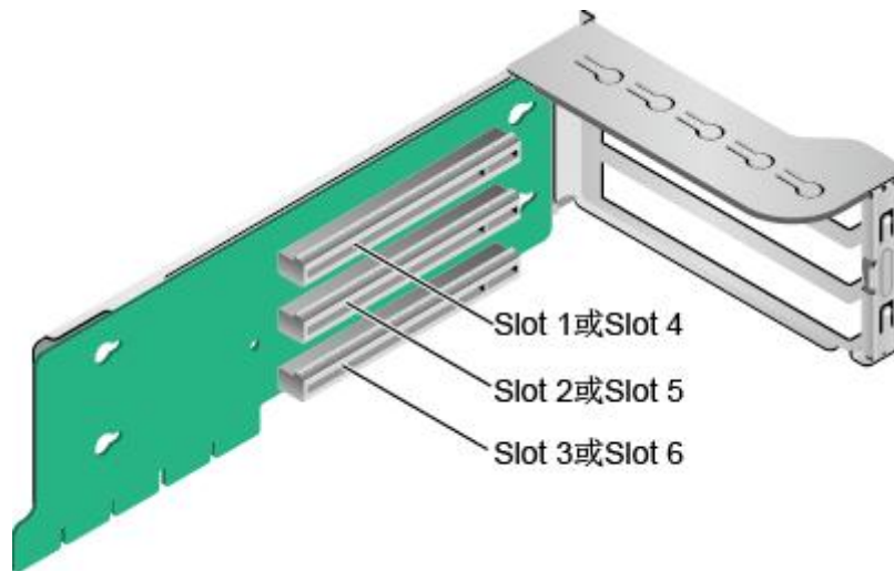
图 4-9 Riser 卡 1 (3x8)
