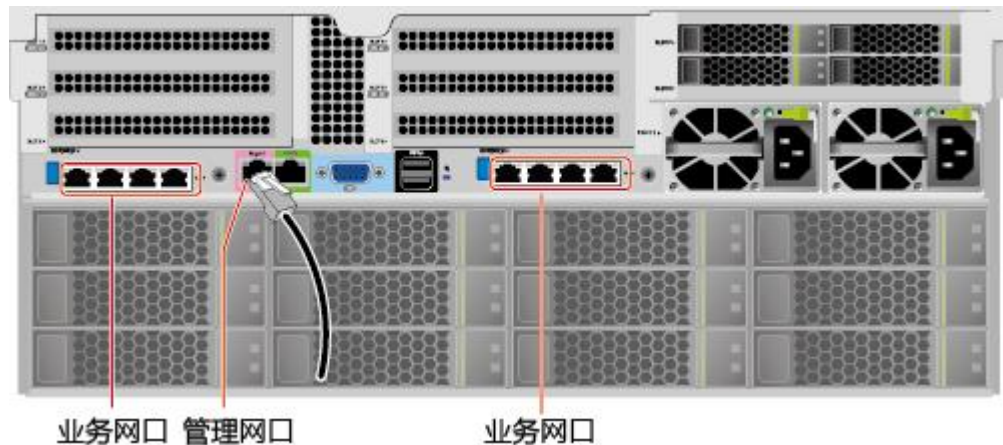
图 6-14 连接网线
