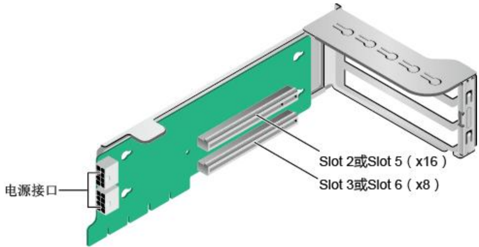
图 3-11 Riser 卡 2 (1x8+1x16)
