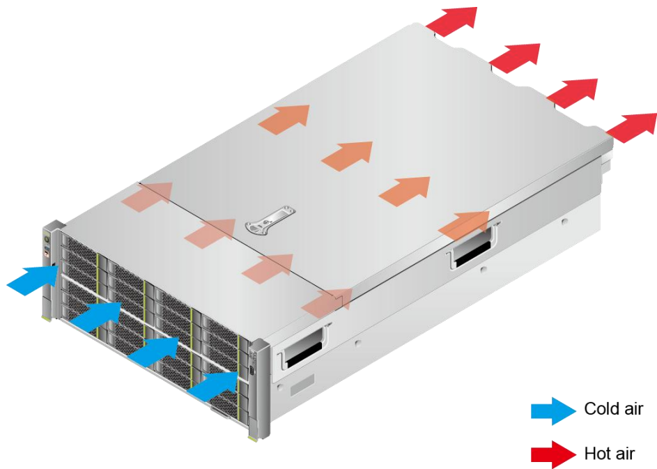
图 6-4 散热气流走向示意图
