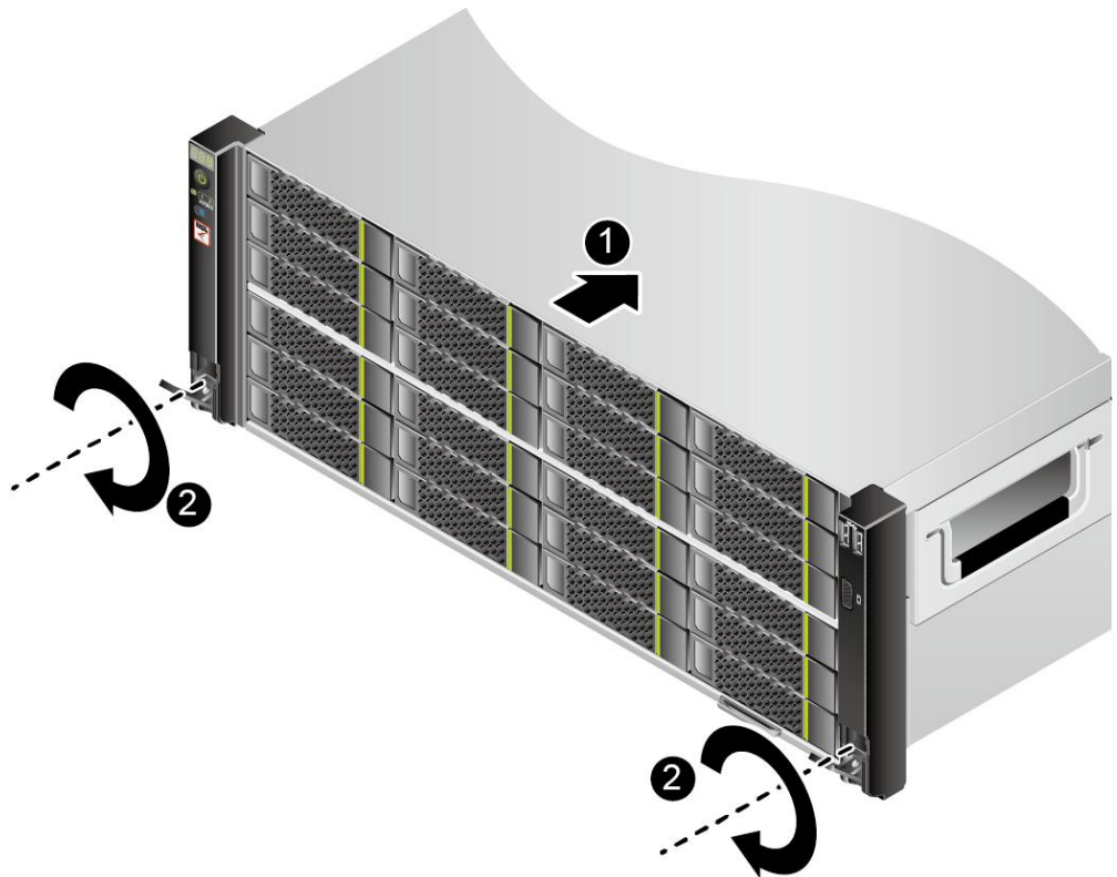
图 6-12 安装服务器
