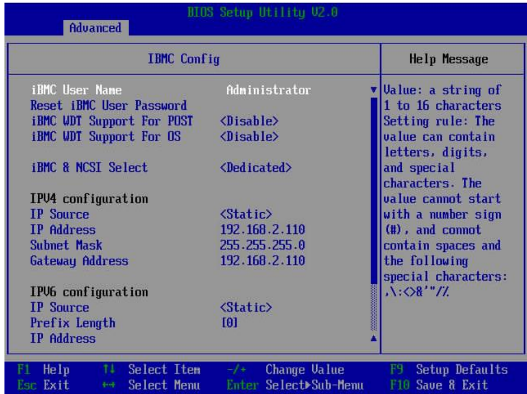
图 6-25 IBMC Config 界面 1
