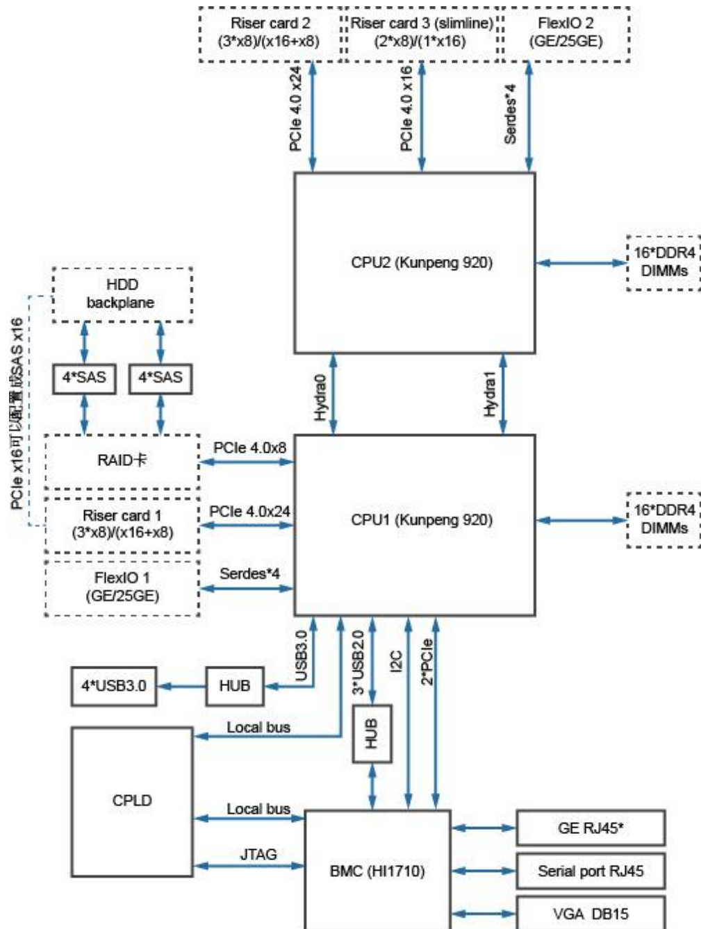
图 2-3 S920X00 (4U) 逻辑结构
