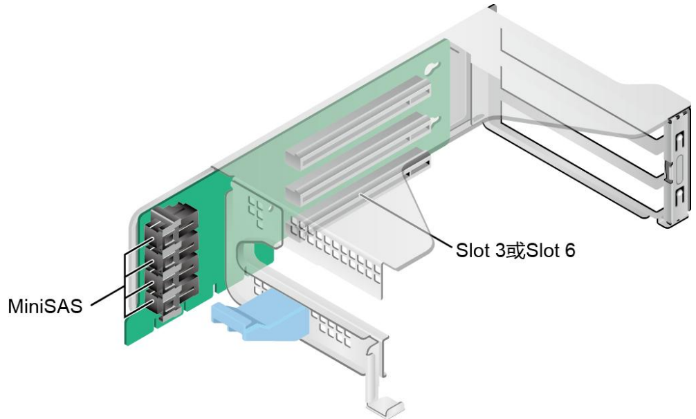
图 3-13 Riser 卡 4 (SAS Riser)
