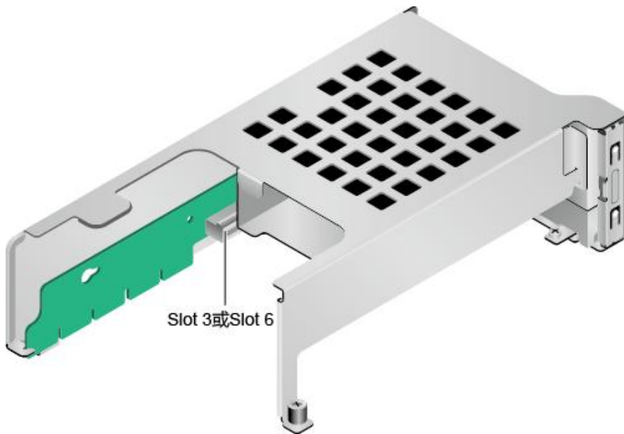
图 3-12 Riser 卡 3 (1x16)
