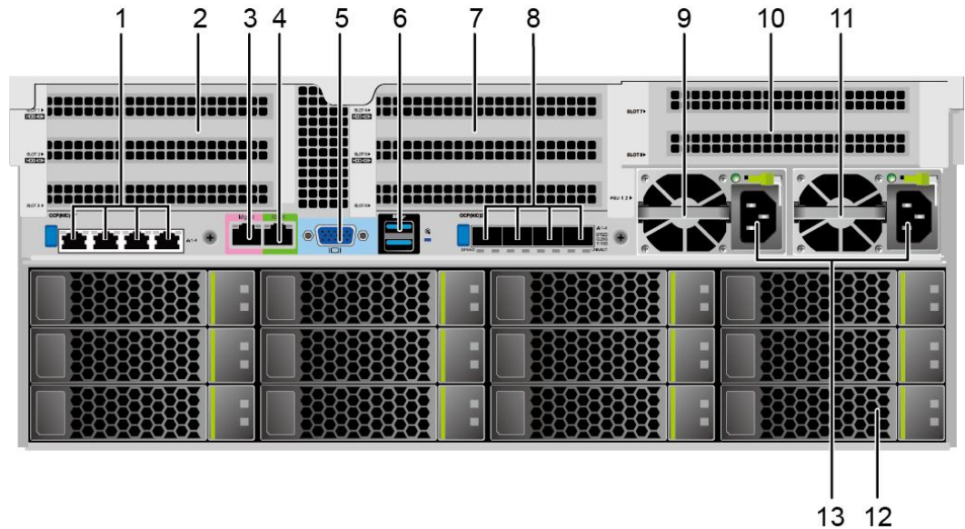
图 3-3 后面板组件
