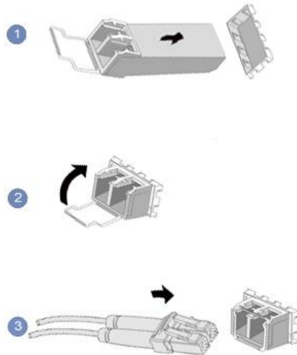
图 6-15 连接光纤
