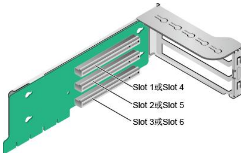
图 3-10 Riser 卡 1 (3x8)
