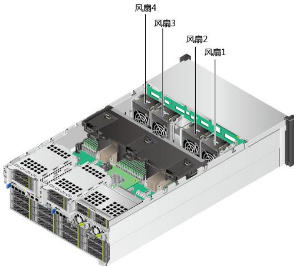
图 3-17 风扇位置图
