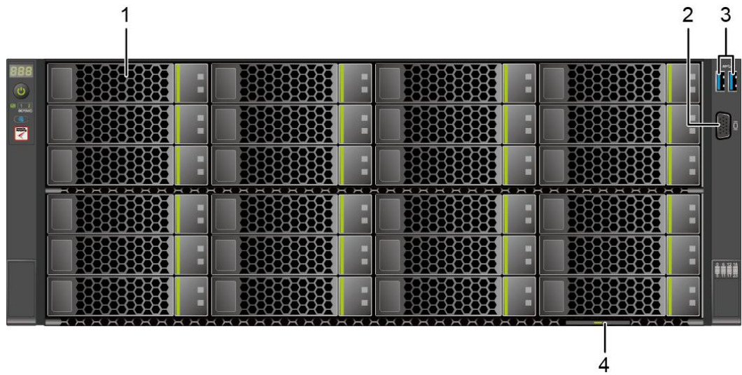
图 3-1 前面板组件
