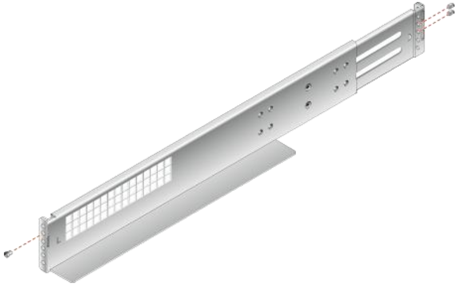
图 6-10 安装限位销钉
