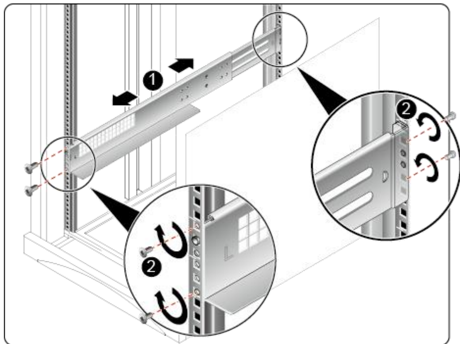
图 6-11 安装可伸缩滑道
