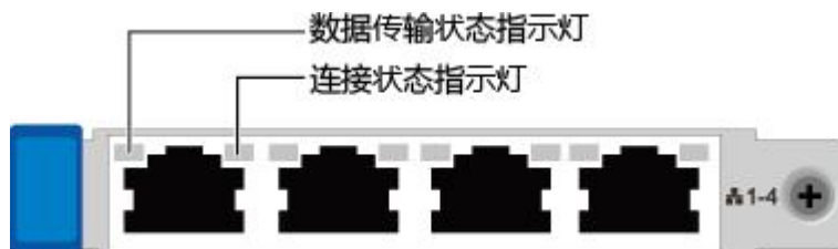
图 3-5 TM210（4xGE 电口）
