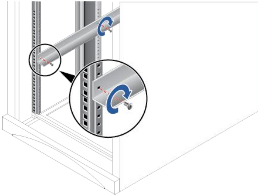
图 6-7 安装 L 型滑道
