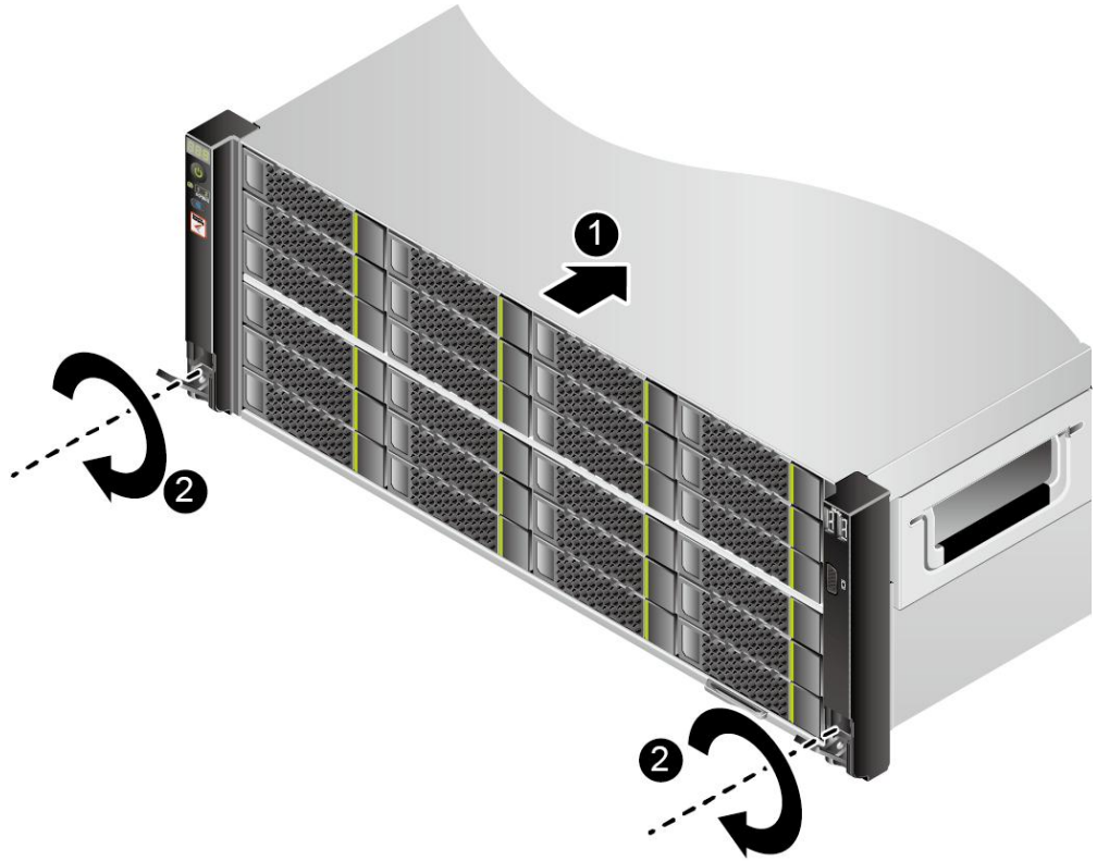
图 6-8 安装服务器
