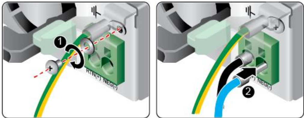
图 6-22 连接线缆
