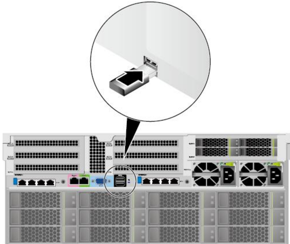
图 6-18 连接 USB 接口
