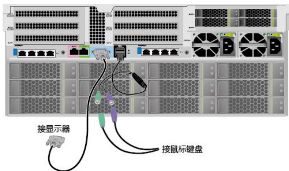
图 6-13 连接 USB 转 PS2 线缆和 VGA 接口
