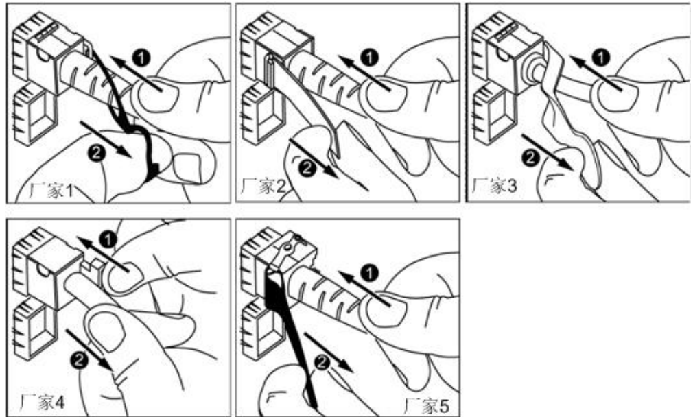
图 6-16 拔出 SFP+ 电缆
