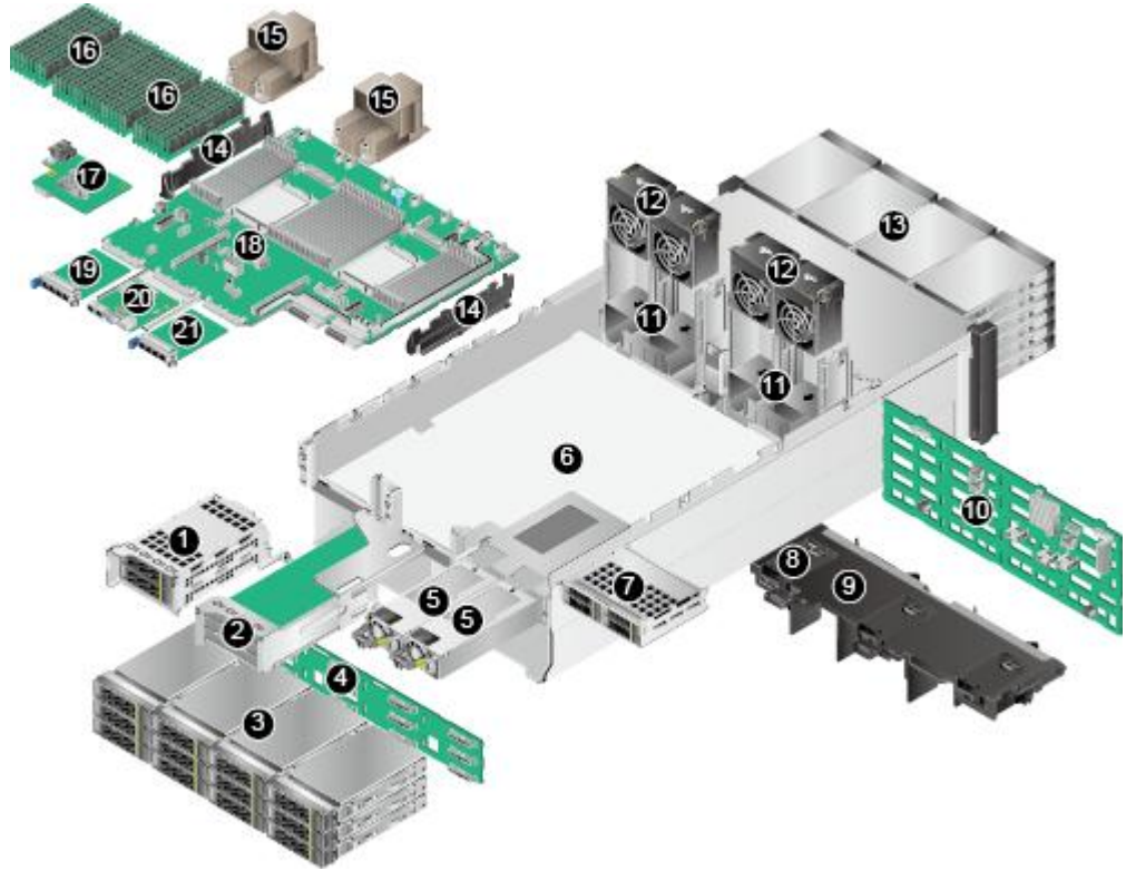
图 2-2 部件
