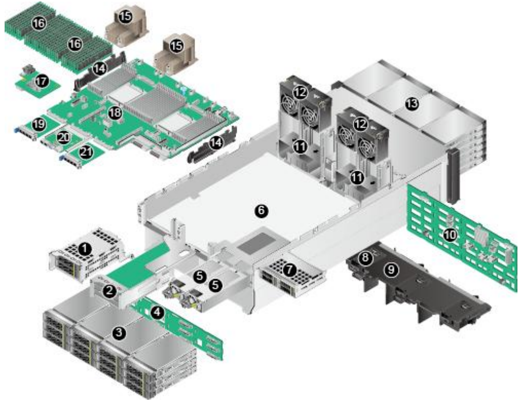
图 4-16 部件
