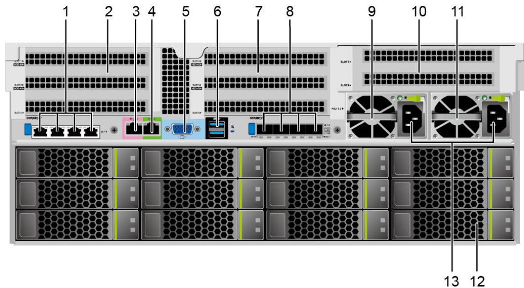
图 4-2 后面板组件
