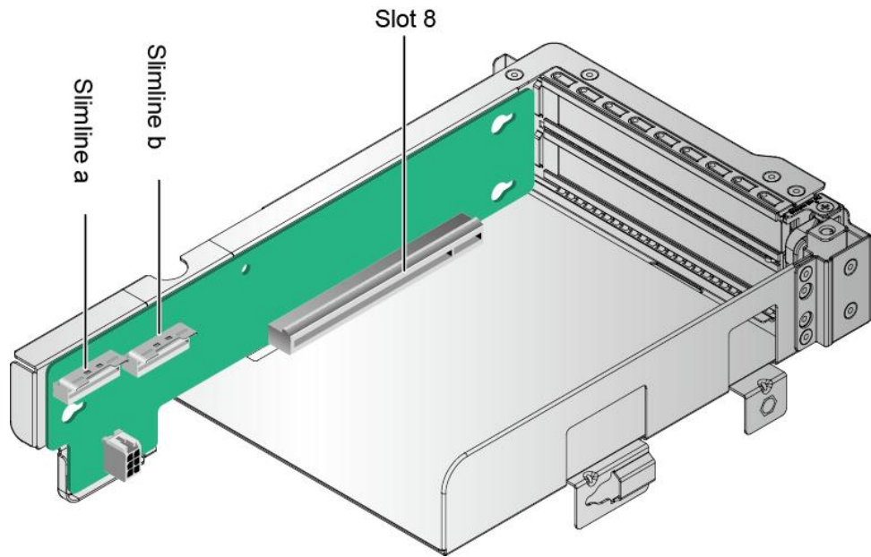
图 4-14 Riser 卡 6 (1x16)
