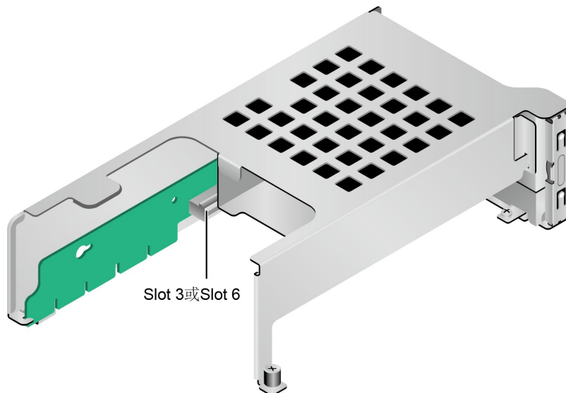
图 2-13 1x16 Riser 卡 3
