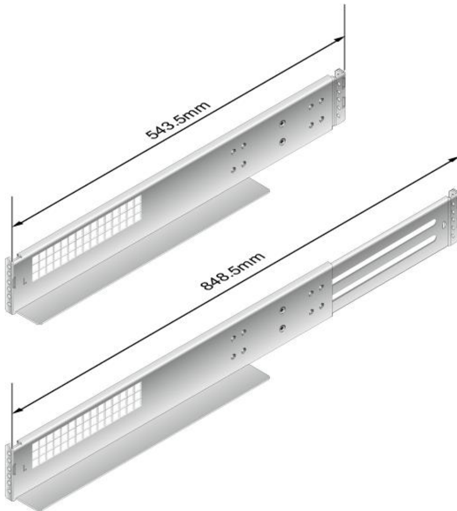
图 5-9 机柜前后方孔条的距离范围
