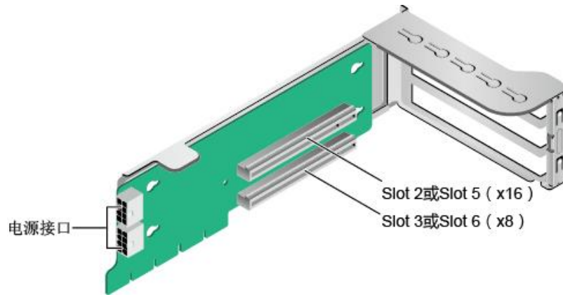
图 2-12 1x8+1x16 Riser 卡 2
