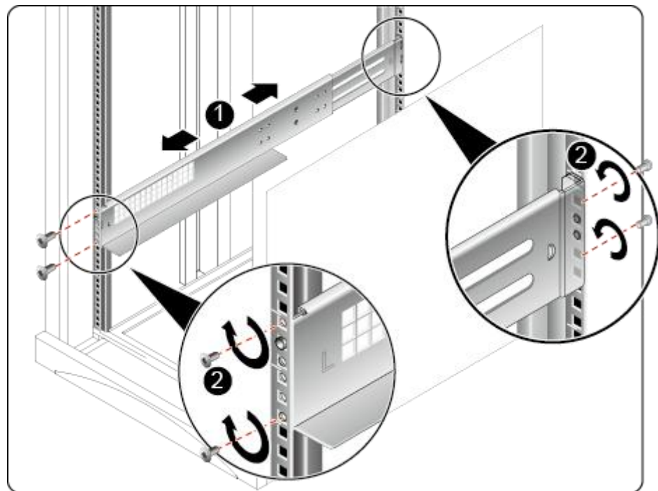
图 5-11 安装可伸缩滑道
