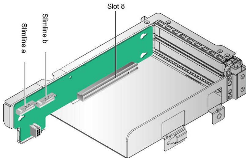
图 2-17 1x16 Riser 卡 7
