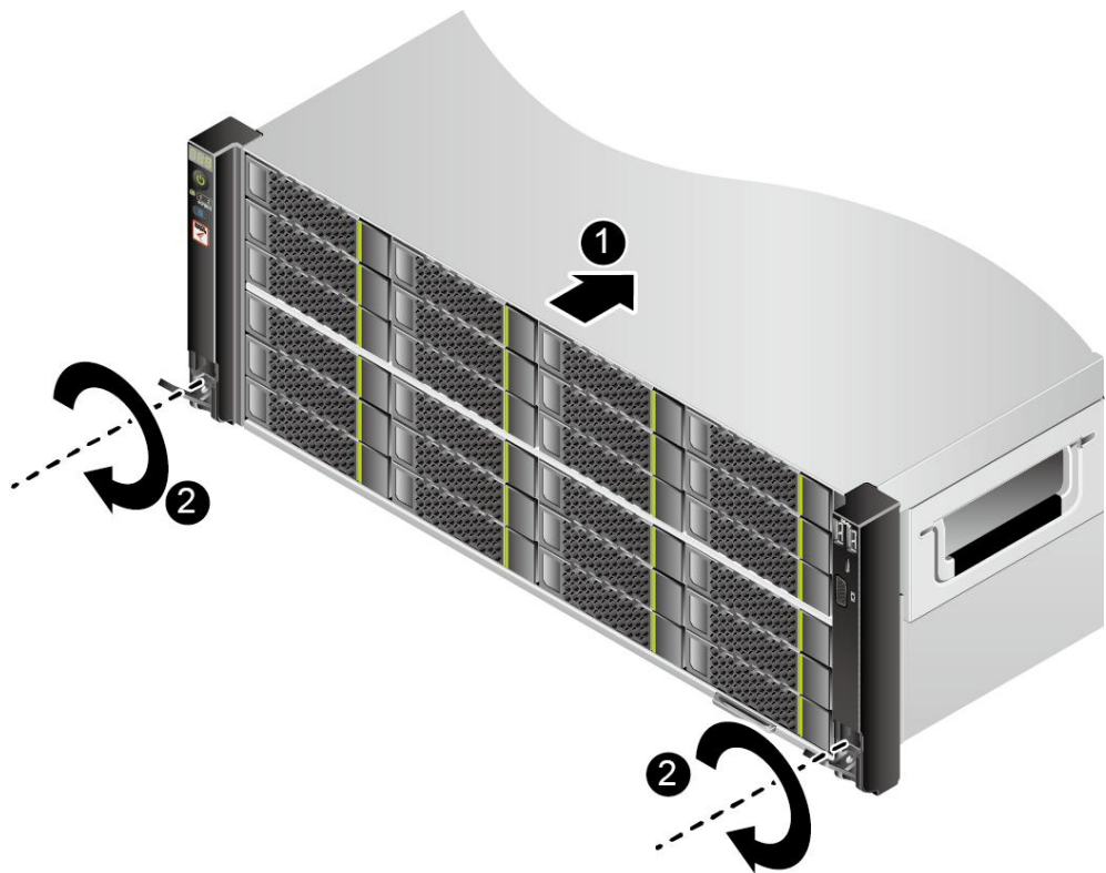
图 5-12 安装服务器
