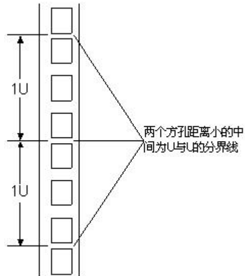
图 5-5 机柜导槽 U 与 U 的间距区分示意图
