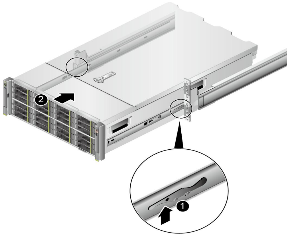
图 5-18 将服务器推入抱轨
