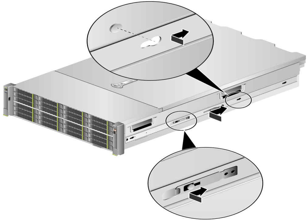
图 5-15 安装内轨
