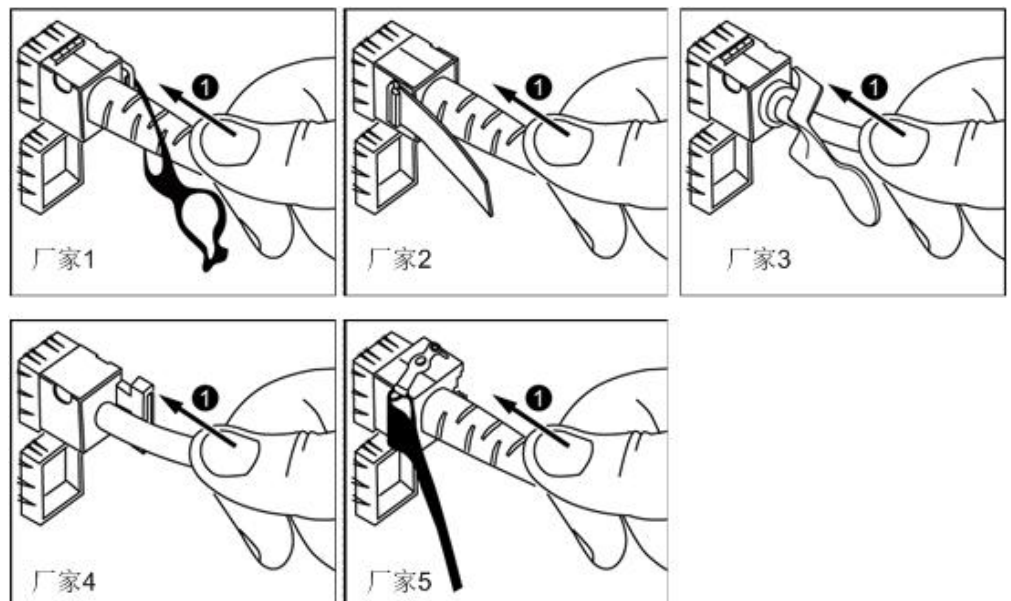
图 5-25 连接 SFP+ 电缆
