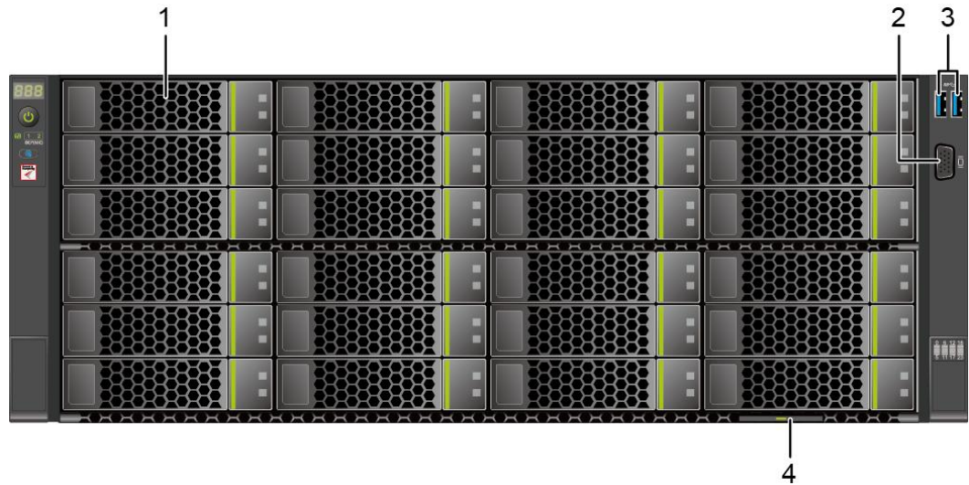
图 2-1 前面板组件
