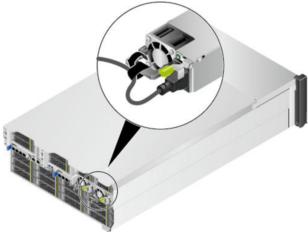
图 5-29 固定电源线缆
