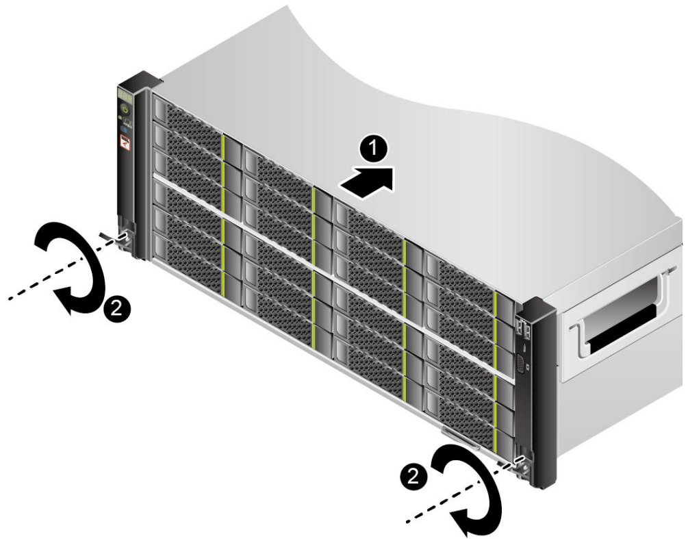
图 5-8 安装服务器
