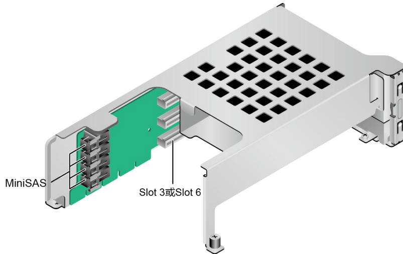
图 2-14 2x2.5 背板 SAS Riser 卡 4
