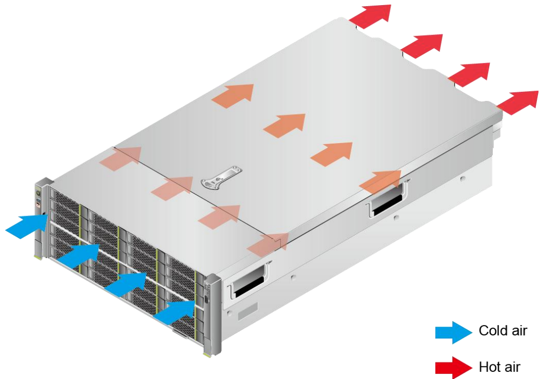
图 5-4 散热气流走向示意图
