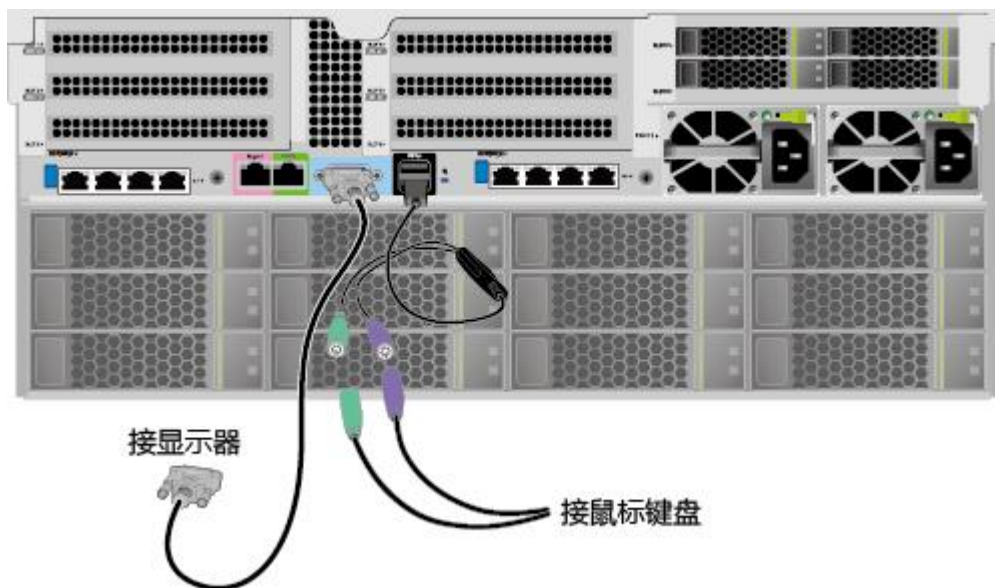
图 5-21 连接 USB 转 PS2 线缆和 VGA 接口
