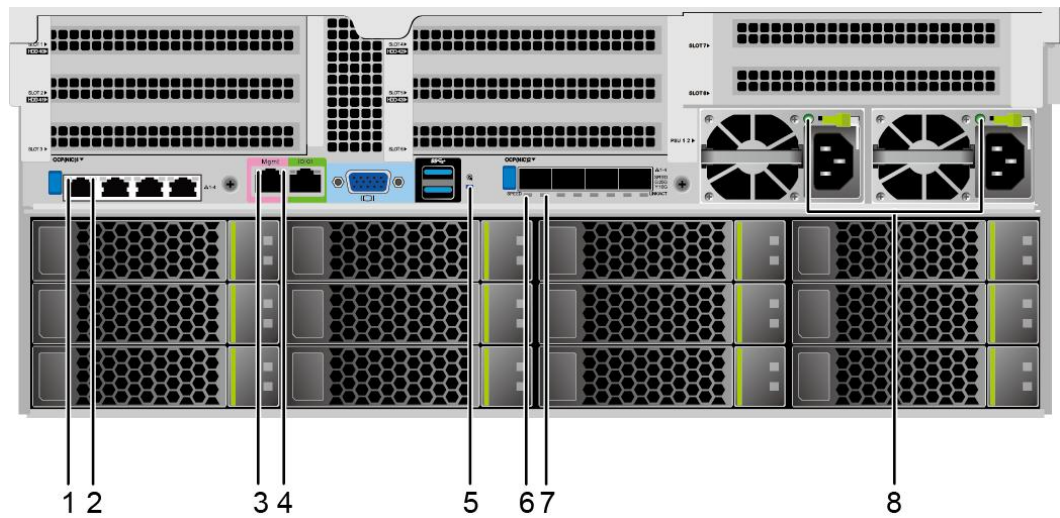
图 2-4 后面板指示灯
