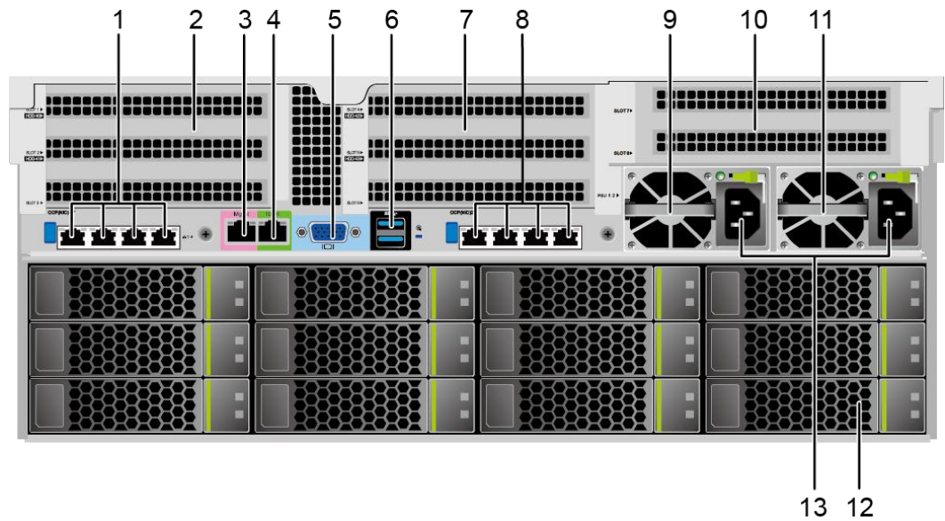
图 2-3 后面板组件
