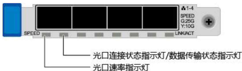
图 2-7 TM280 (4*25GE 光口)
