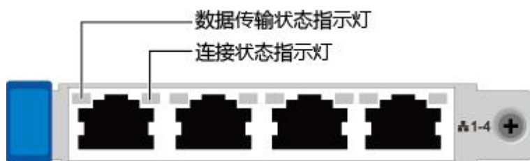
图 2-5 TM210（4*GE 电口）
