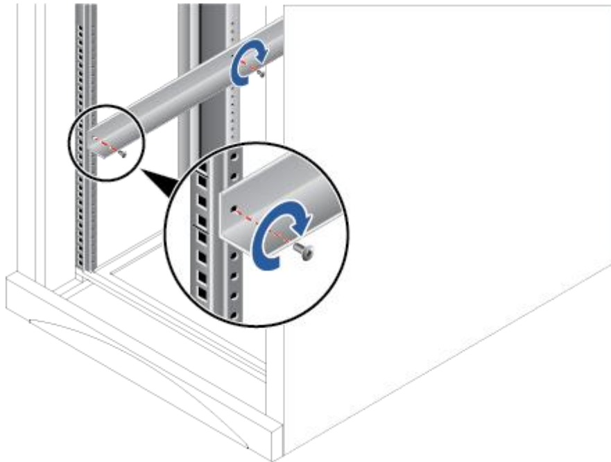
图 5-7 安装 L 型滑道
