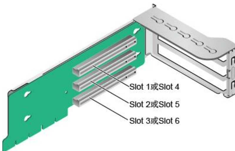
图 2-11 3x8 Riser 卡 1
