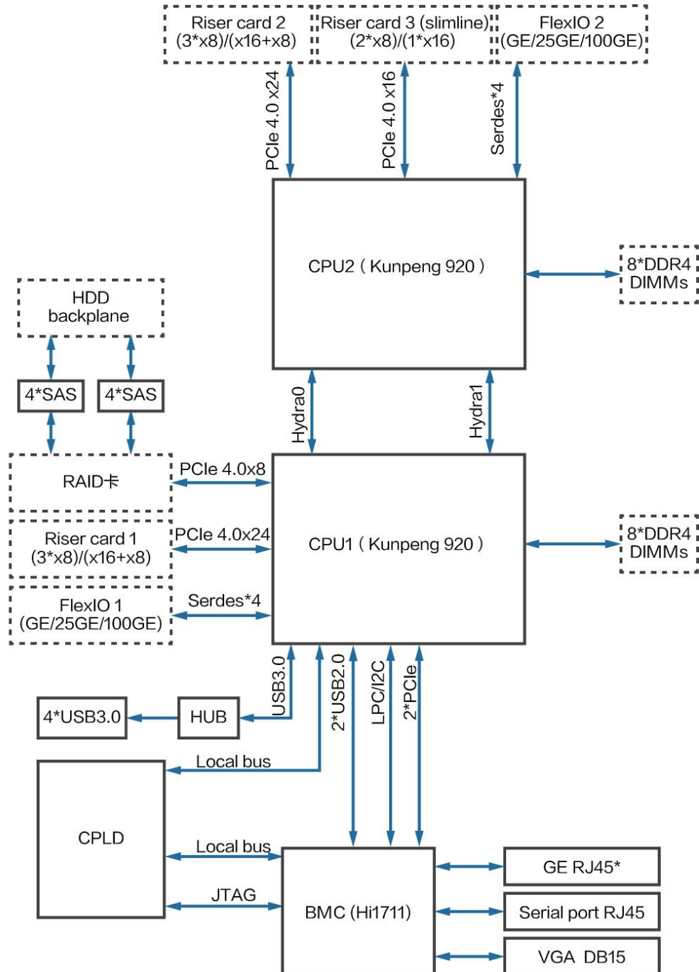
图 1-3 服务器逻辑结构
