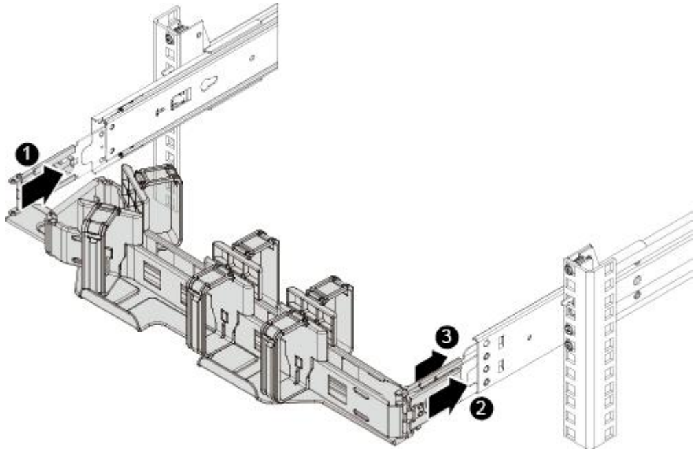
图 5-20 安装理线架
