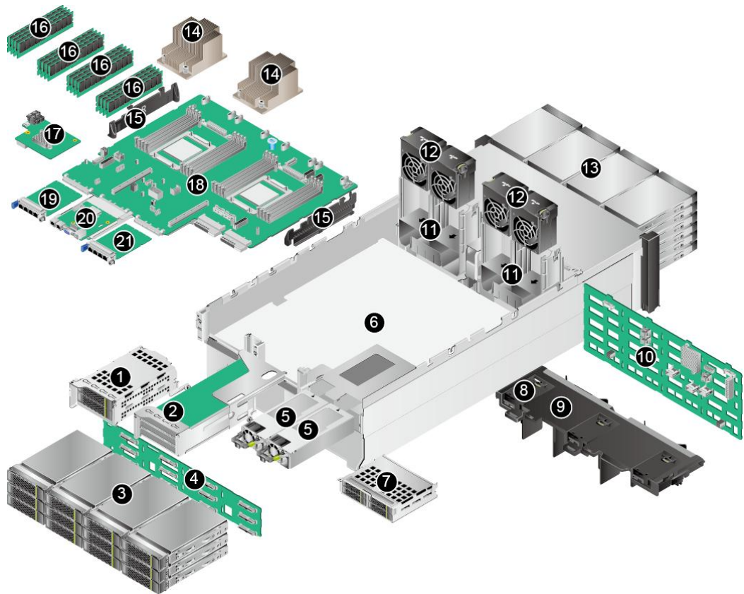
图 1-2 部件
