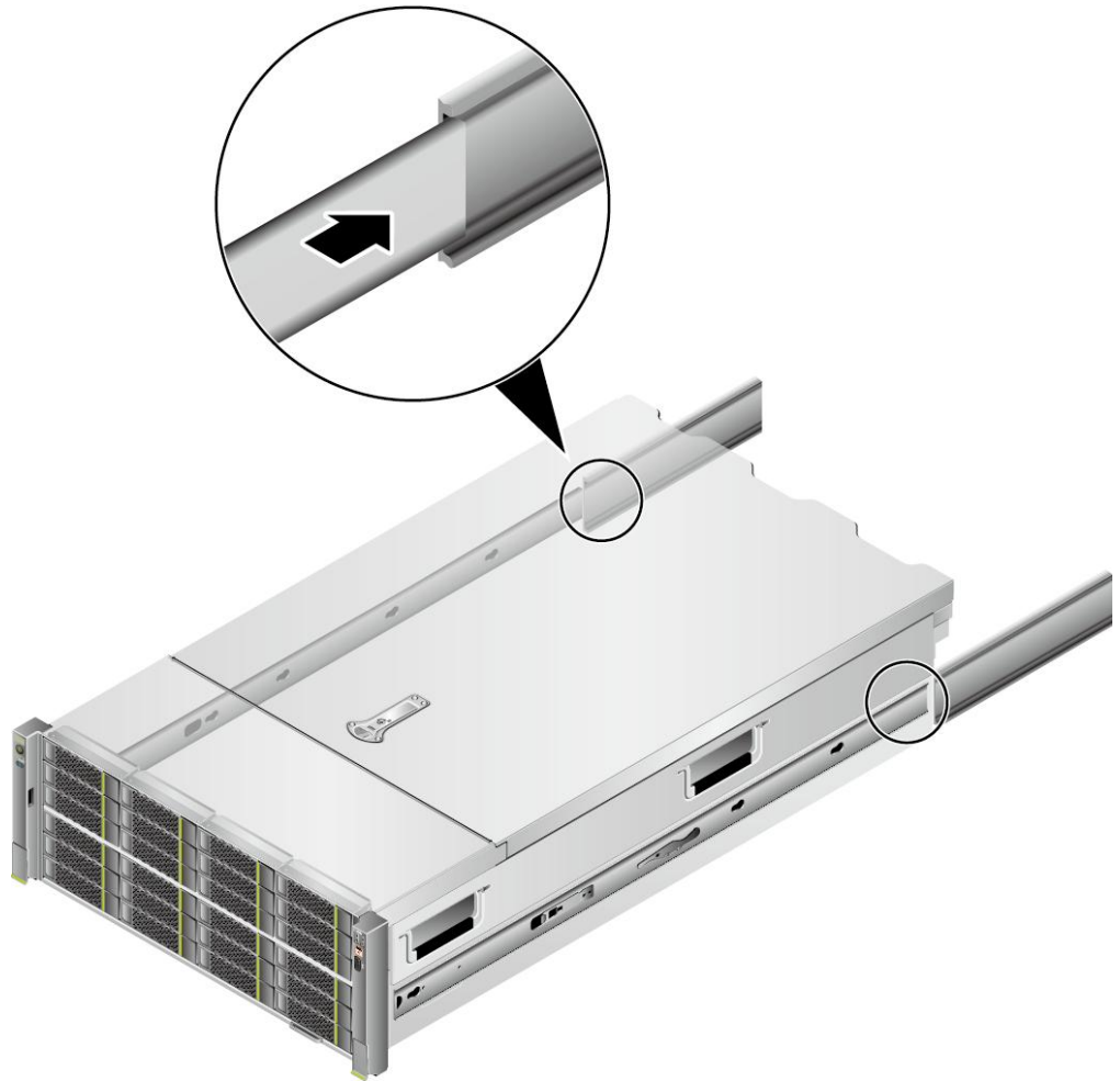
图 5-16 安装服务器
