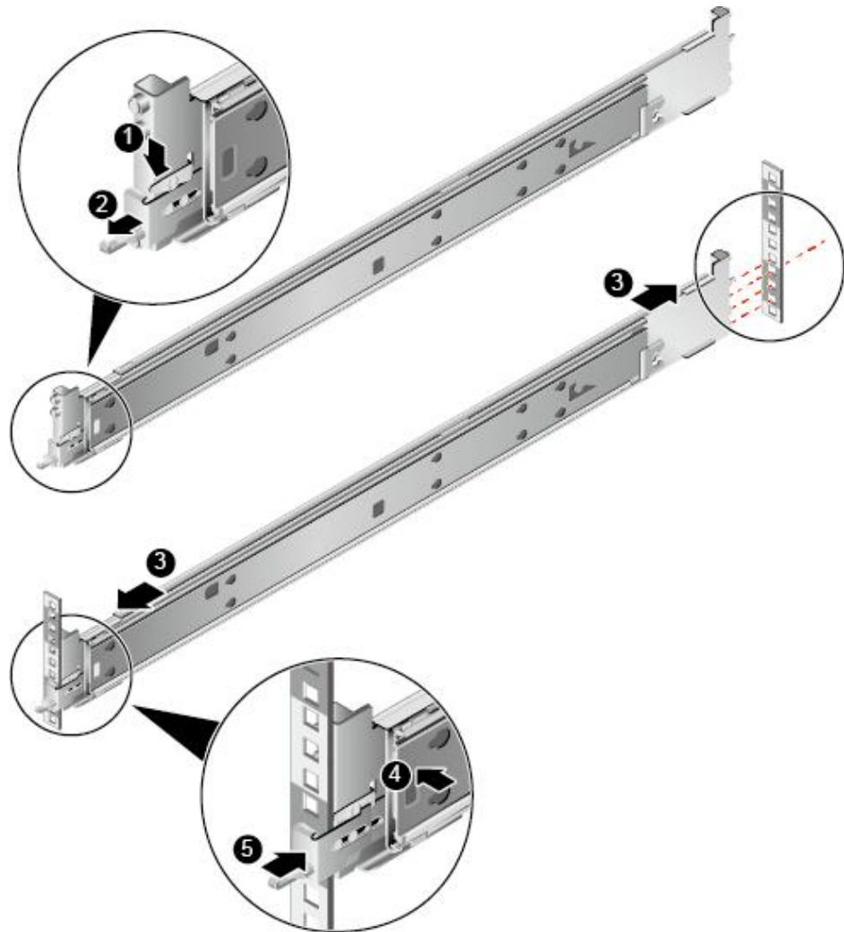
图 5-13 安装抱轨前后端
