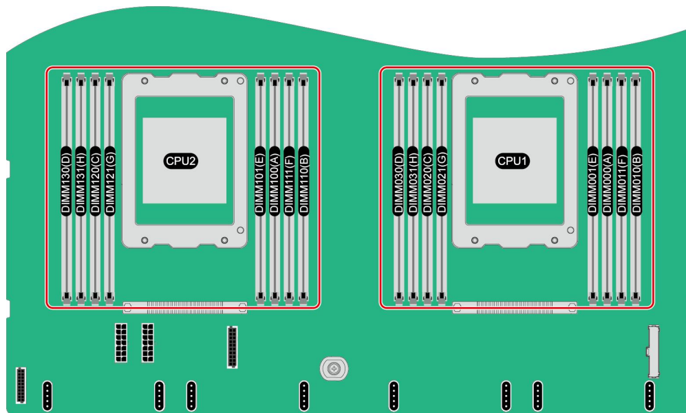
图 4-1 内存槽位编号
