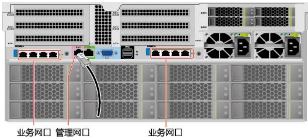
图 5-22 连接网线
