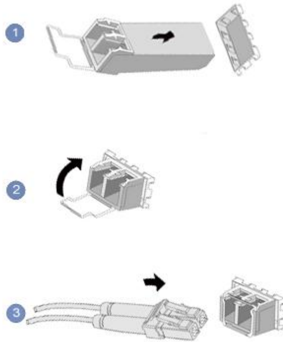
图 5-23 连接光纤
