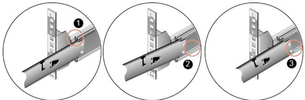
图 5-17 将内轨卡入塑胶卡槽
