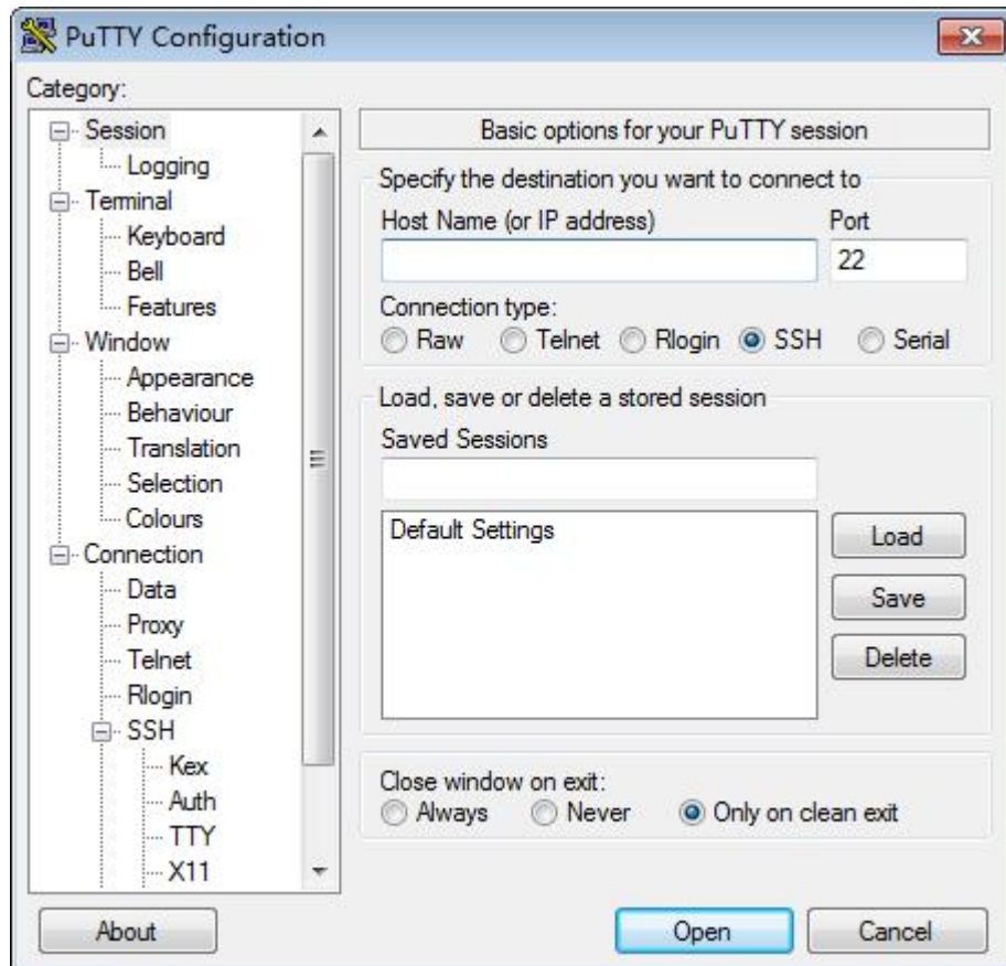
图 7-16 PuTTY Configuration
