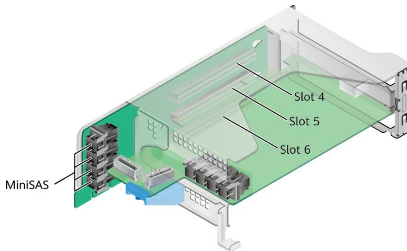
图 2-15 IOB 卡 SAS Riser 卡 5
