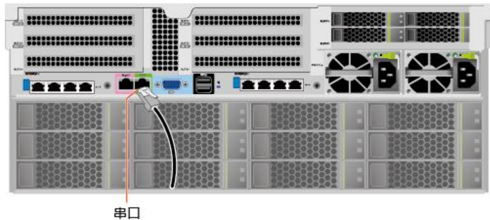
图 5-27 连接串口线缆
