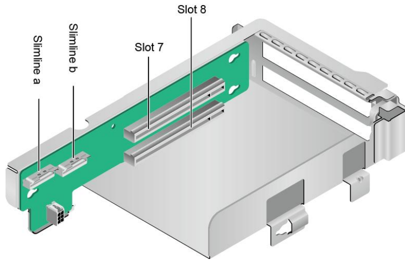
图 2-16 2x8 Riser 卡 6
