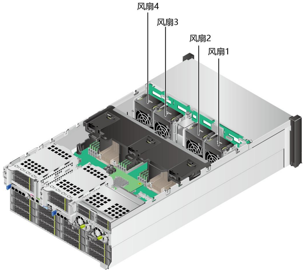
图 2-19 风扇位置图
