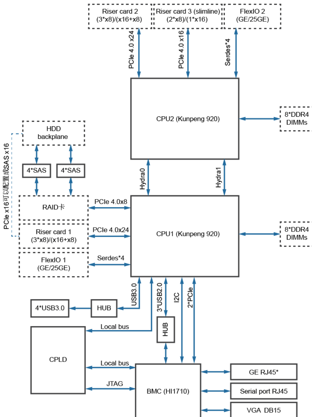
图 2-3 服务器逻辑结构
