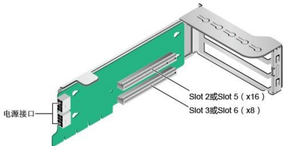
图 3-15 Riser 卡 2 (1x8+1x16)
