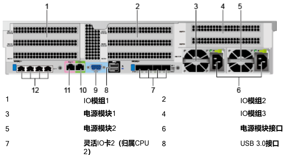
后面板组件
