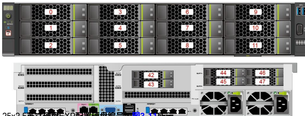
图 3-10 12x3.5 英寸硬盘直通配置
