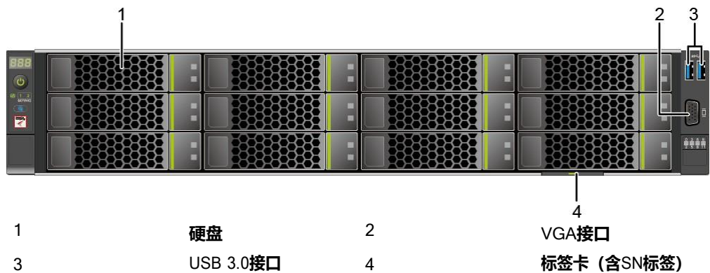
图 3-1 12x3.5 英寸硬盘配置前面板组件
