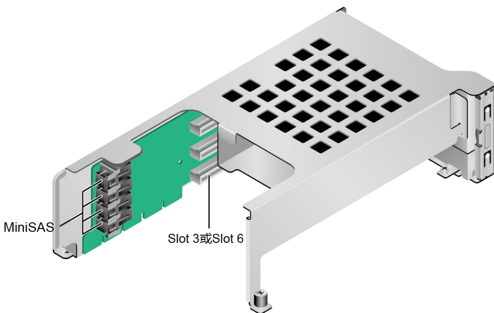
图 3-17 Riser 卡 5 (SAS Riser)
