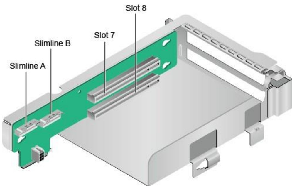
图 3-18 Riser 卡 6 (2x8)
