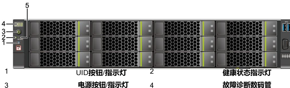
图 3-3 12x3.5 英寸硬盘配置前面板指示灯和按钮
