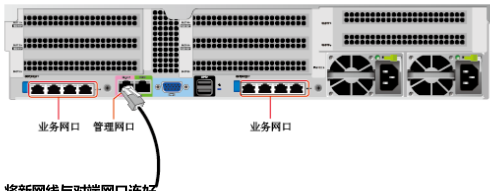
图 6-11 连接网线
