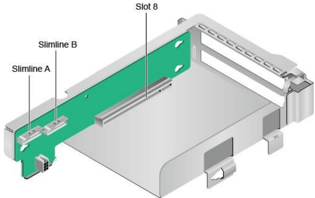
图 3-19 Riser 卡 7 (1x16)
