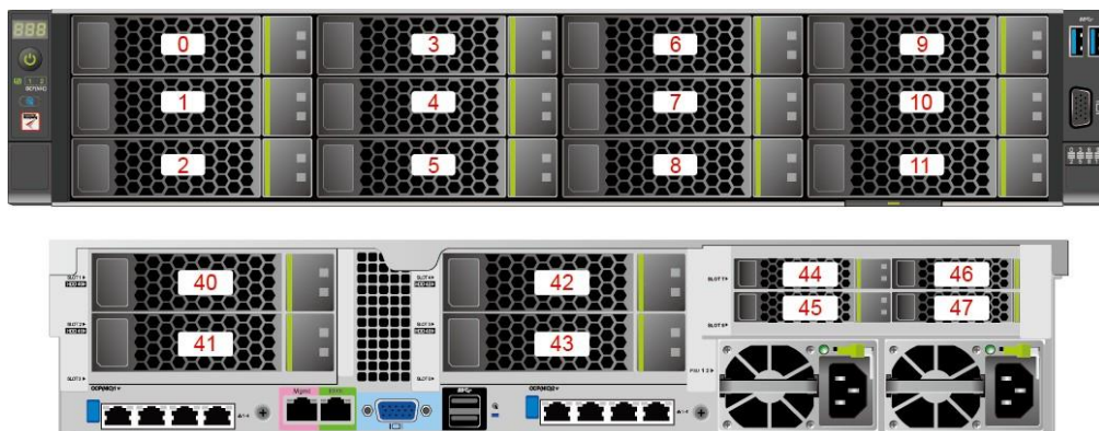
图 3-9 12x3.5 英寸硬盘 EXP 配置硬盘编号
