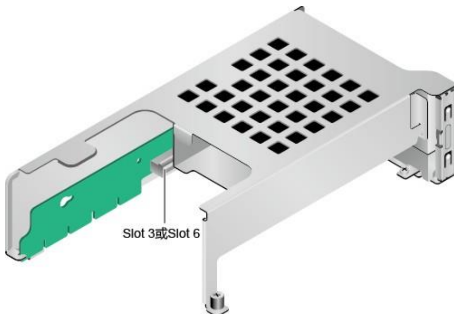
图 3-16 Riser 卡 4 (1x16)
