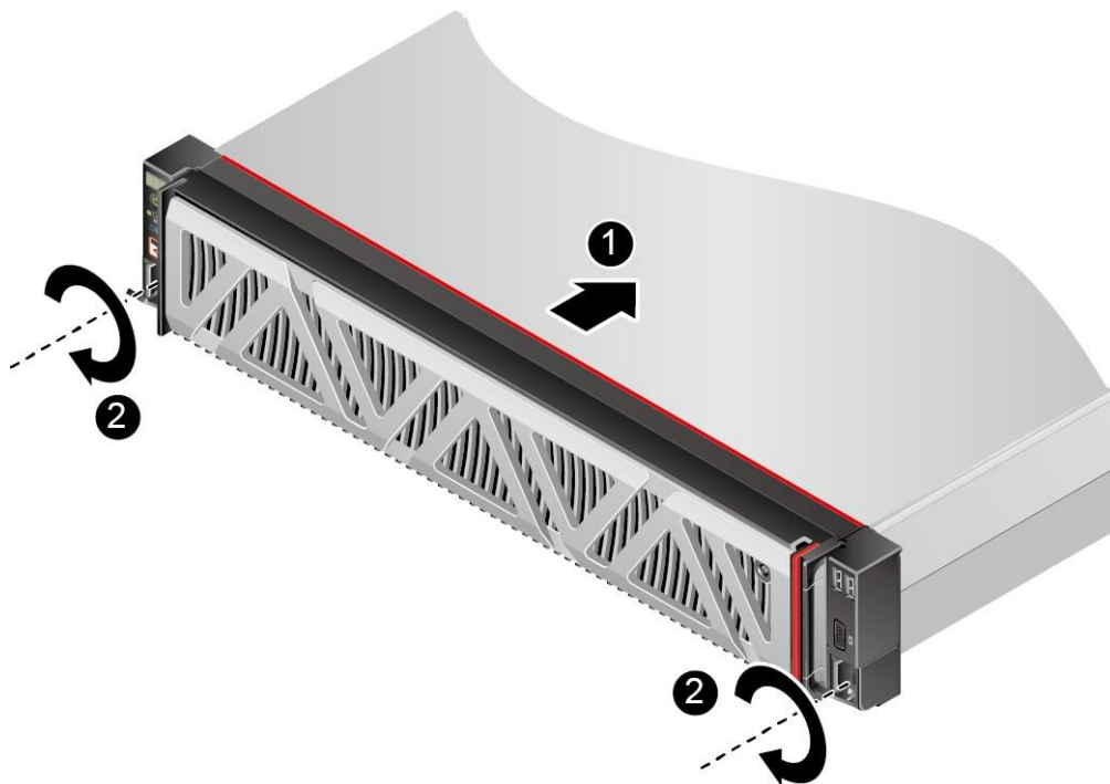
图 6-9 安装服务器
