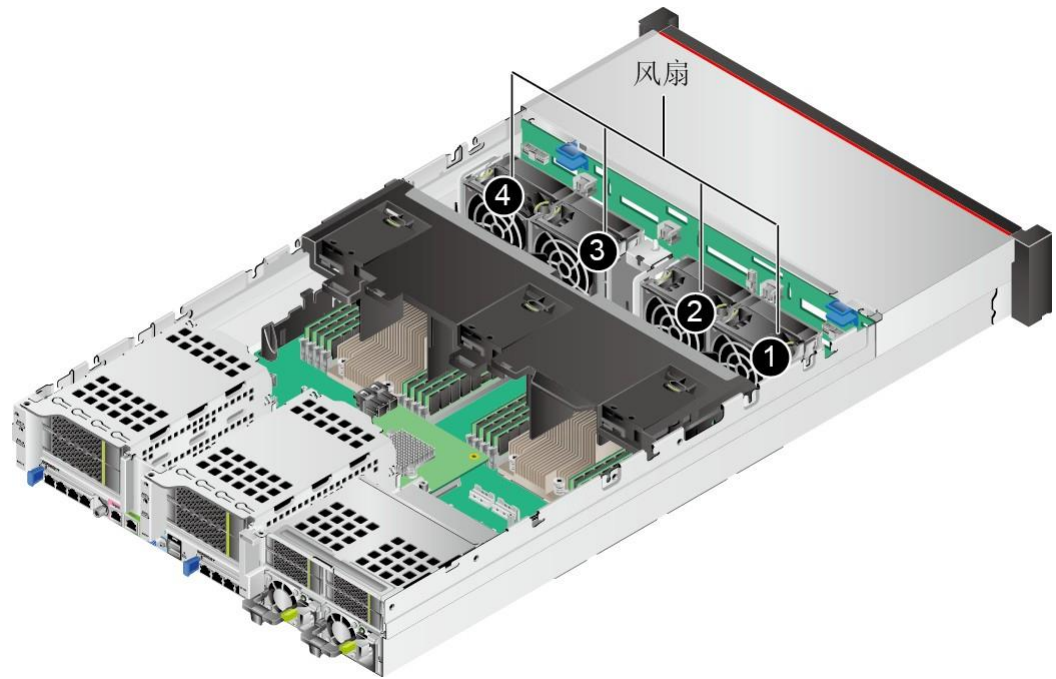
图 3-21 风扇位置图
