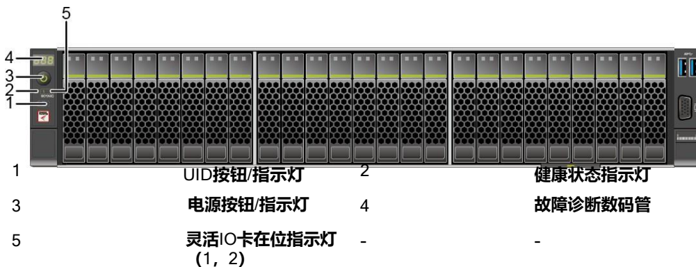
图 3-4 25x2.5 英寸硬盘配置前面板指示灯和按钮
