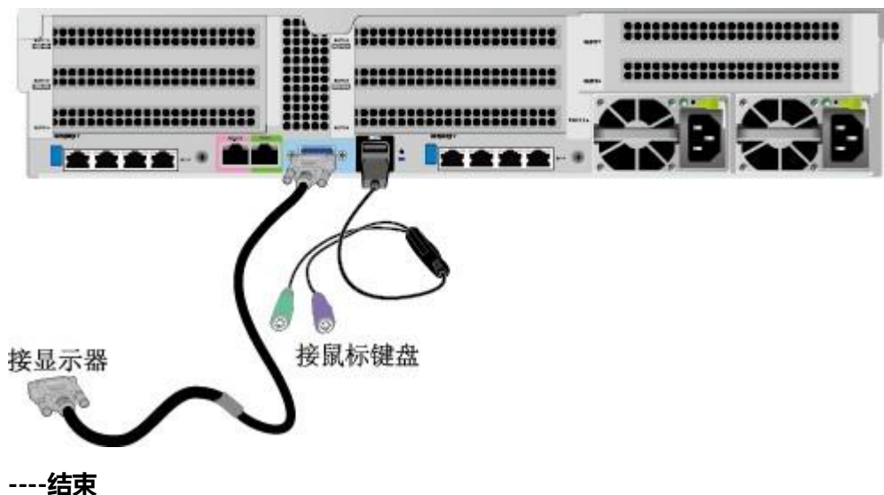
图 6-10 连接 USB 转 PS2 线缆和 VGA 接口
