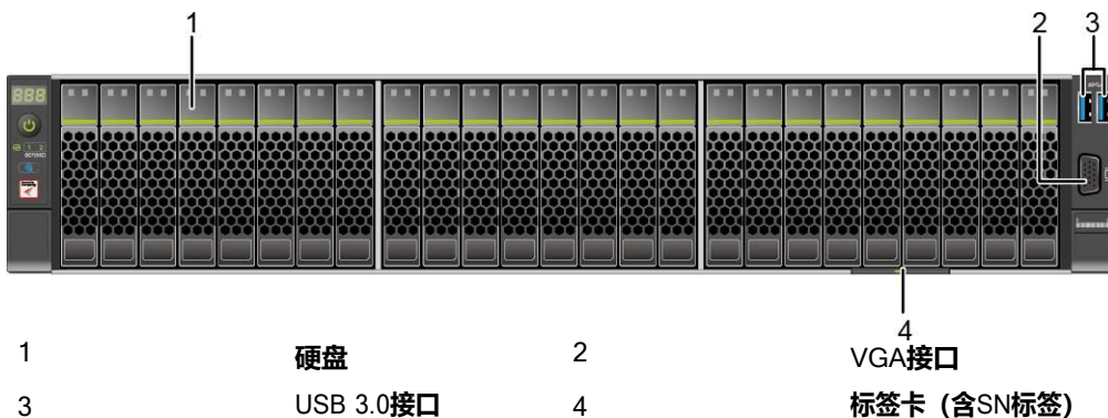
图 3-2 25x2.5 英寸硬盘配置前面板组件
