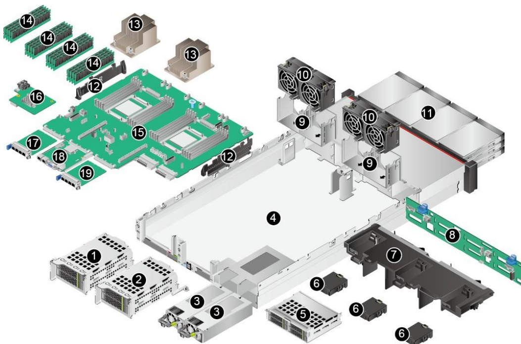
图 2-2 部件
