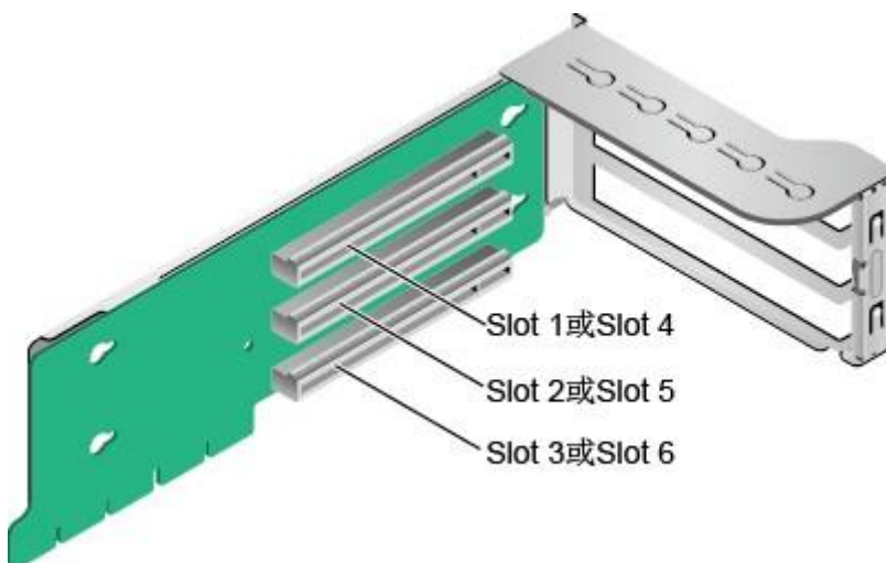
图 3-14 Riser 卡 1 (3x8)
