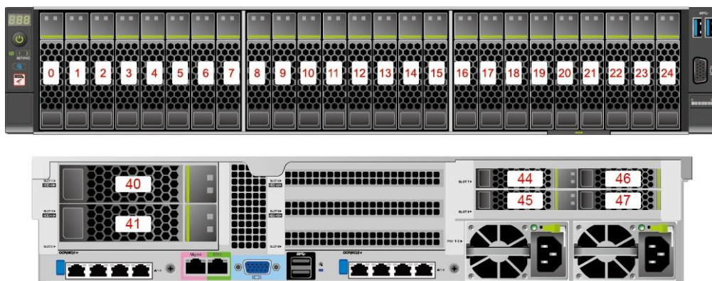
图 3-11 25x2.5 英寸硬盘 EXP 配置硬盘编号
