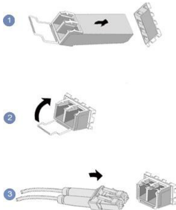
图 6-12 连接光纤
