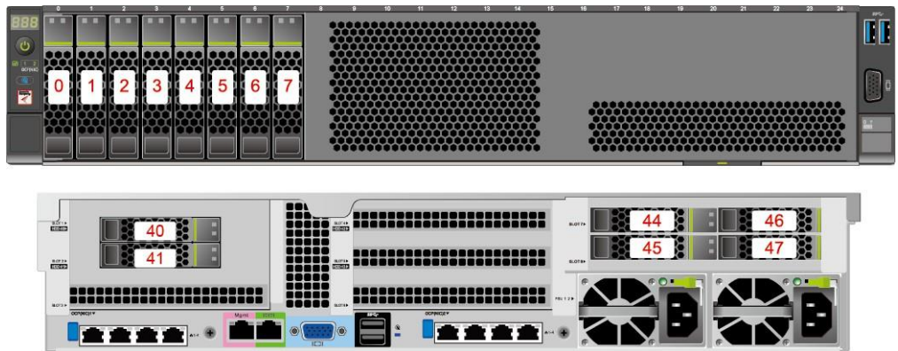
图 3-26 8x2.5 英寸硬盘直通配置的硬盘编号
