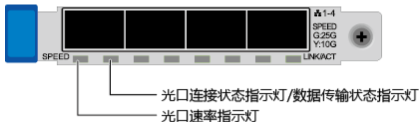
图 3-16 TM280 ( 4*25GE 光口 )
