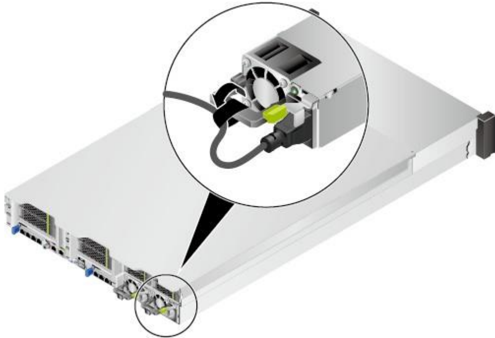
图 6-18 固定电源线缆
