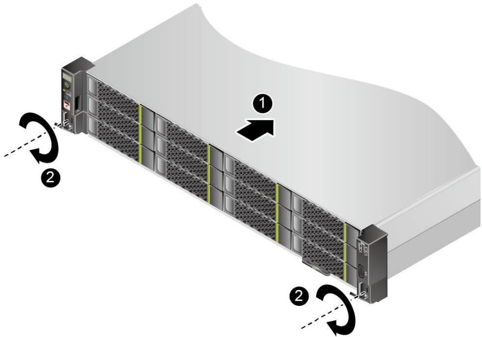
图 6-9 安装服务器
