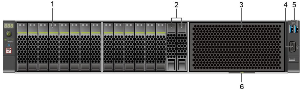
图 3-5 8x2.5 SAS/SATA+6x2.5 NVMe 硬盘配置前面板组件
