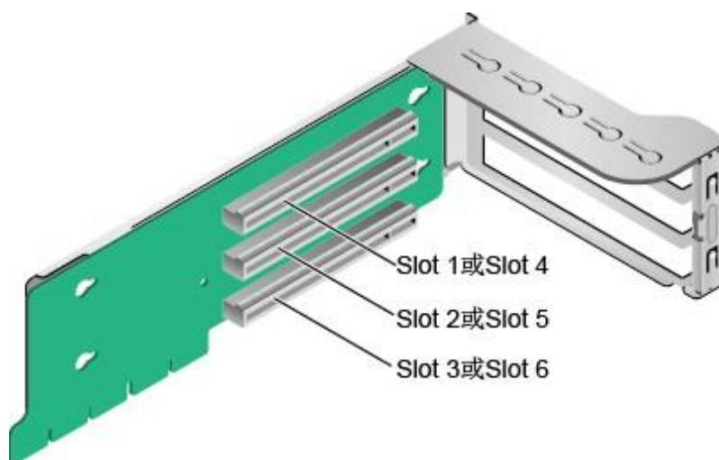
图 3-29 Riser 卡 1 ( 3x8 )
