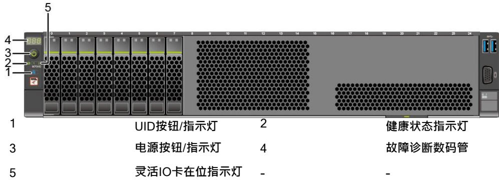
图 3-12 8x2.5 英寸硬盘配置前面板指示灯和按钮
