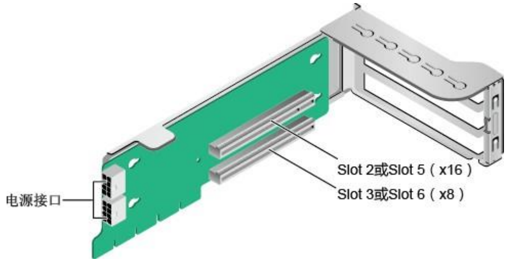
图 3-30 Riser 卡 2 ( 1x8+1x16 )
