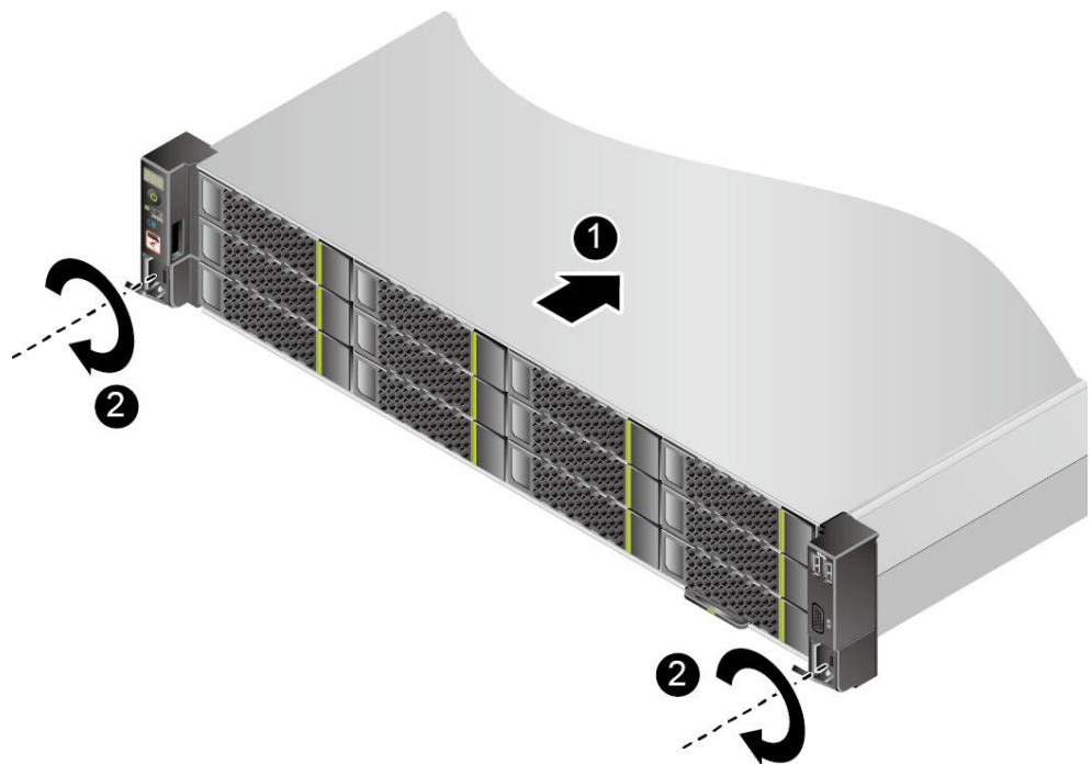
图 6-7 安装服务器
