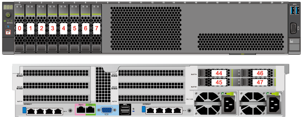
图 3-25 8x2.5 英寸硬盘配置的硬盘编号
