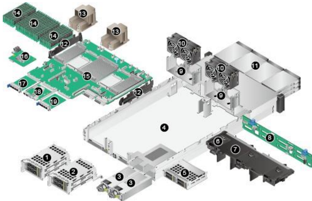
图 2-2 部件
