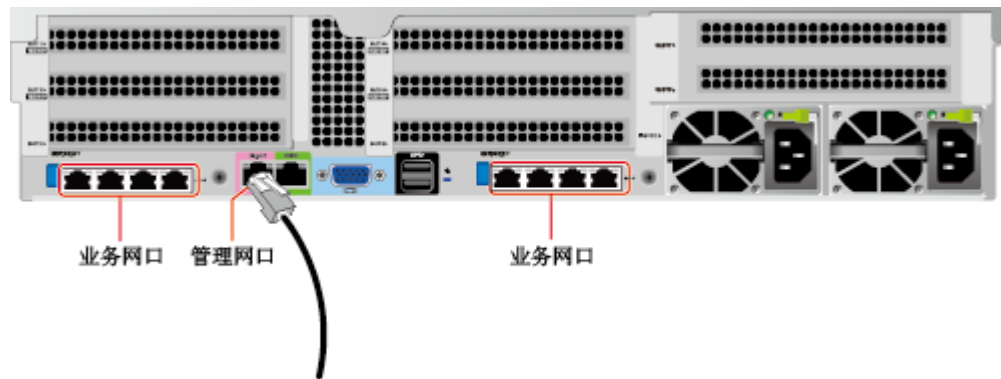
图 6-11 连接网线
