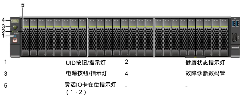
图 3-8 25x2.5 英寸硬盘配置前面板指示灯和按钮
