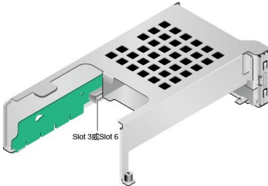
图 3-34 Riser 卡 5 ( 1x16 )
