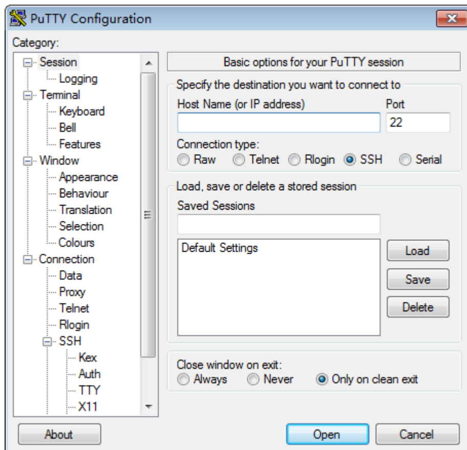
图 8-16 PuTTY Configuration
