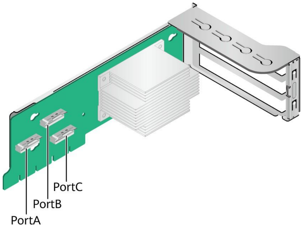
图 3-32 Riser 卡 4
