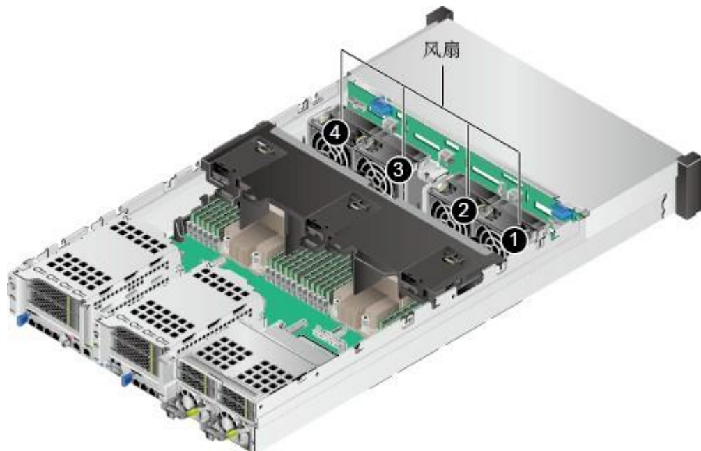
图 3-39 风扇位置图
