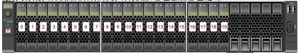
图 3-23 8x2.5 SAS/SATA+12x2.5 NVMe 硬盘配置硬盘编号
