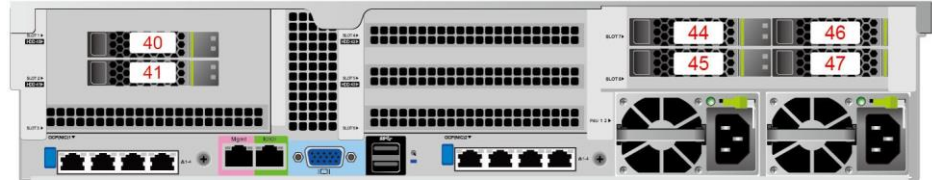
图 3-23 8x2.5 SAS/SATA+12x2.5 NVMe 硬盘配置硬盘编号
