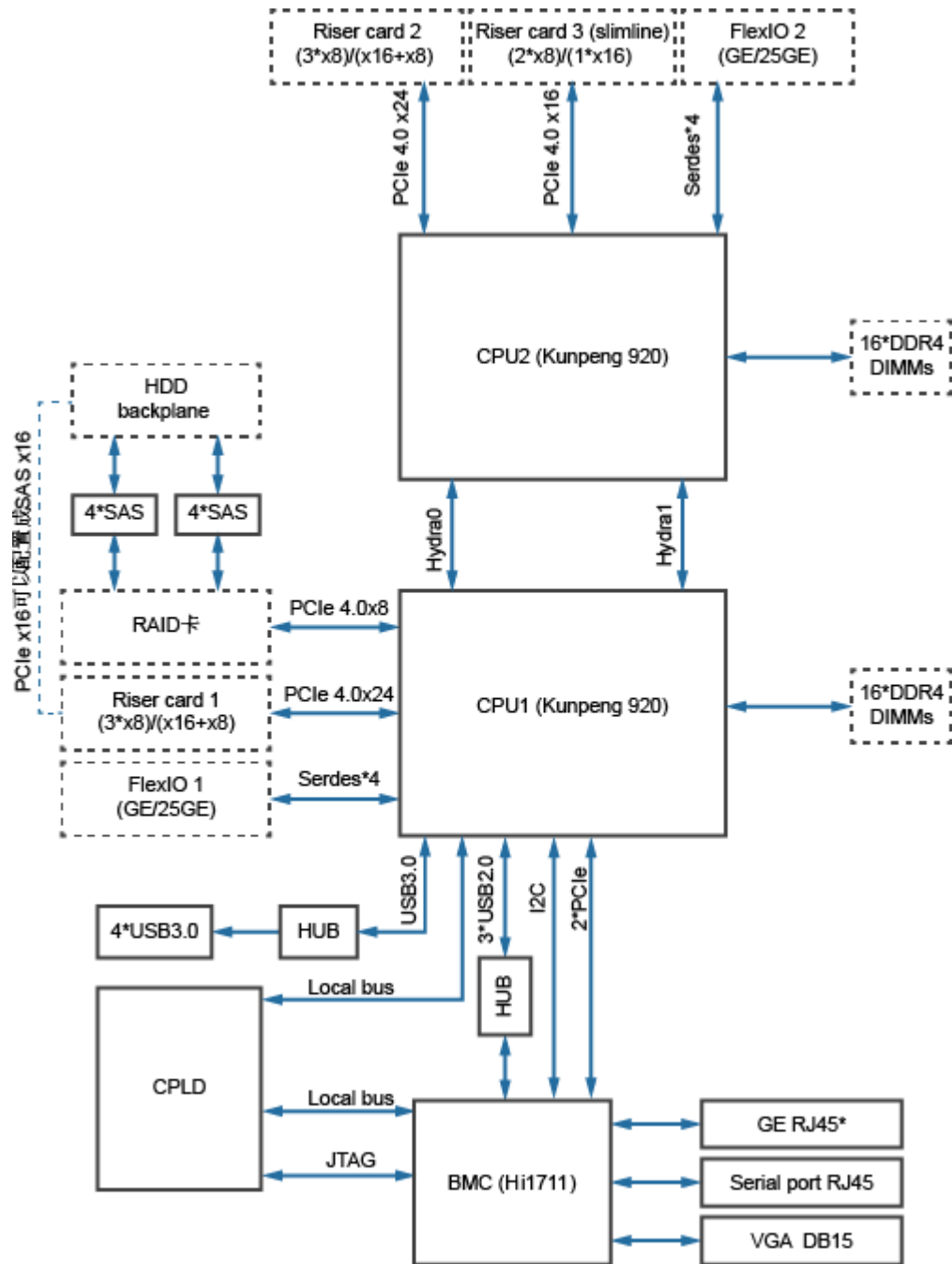
图 2-3 PR210K逻辑结构
