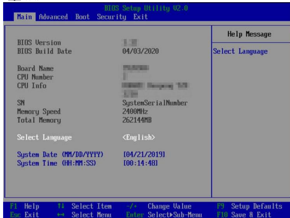
图 6-40 “Main” 界面
