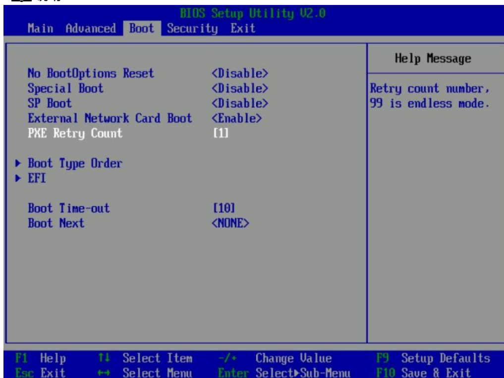
图 6-34 Boot 界面
