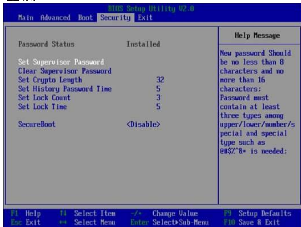
图 6-39 “Security” 界面
