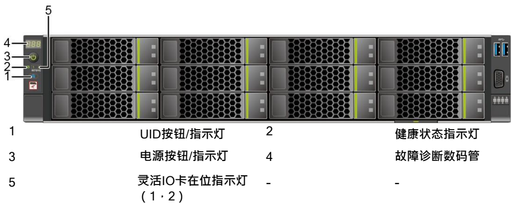
图 3-7 12x3.5 英寸硬盘配置前面板指示灯和按钮
