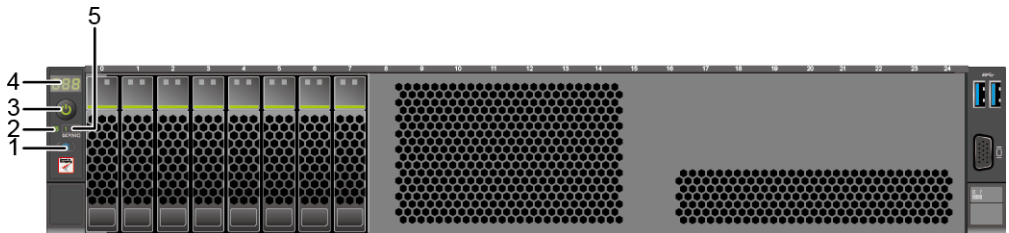
图 3-11 8x2.5 英寸硬盘配置前面板指示灯和按钮
