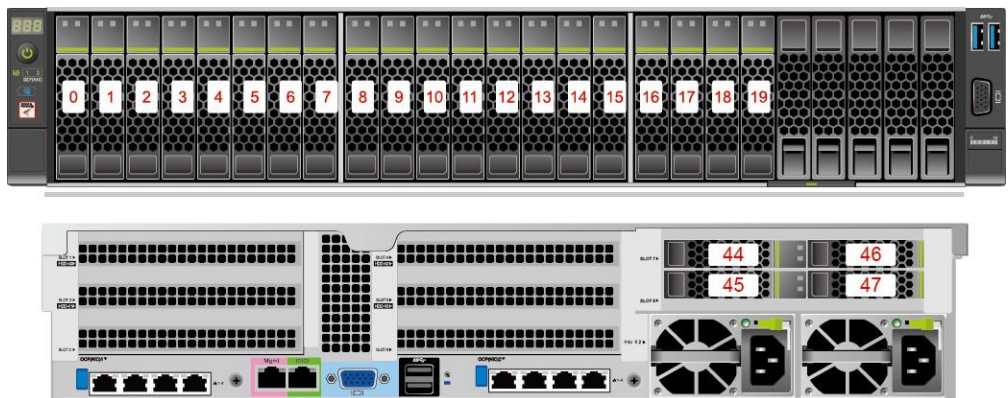
图 3-22 8x2.5 SAS/SATA+12x2.5 NVME 硬盘配置
