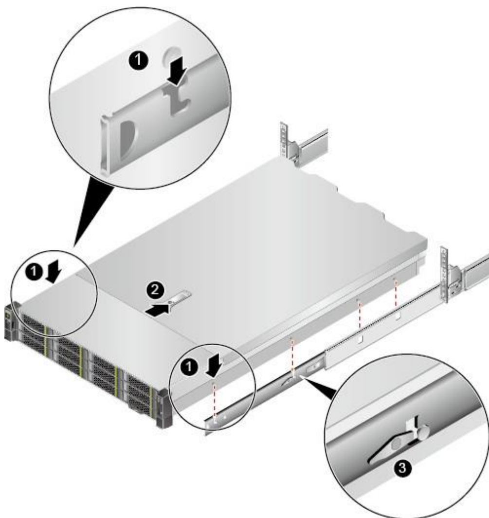
图 6-12 安装服务器
