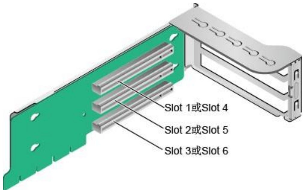
图 3-29 3x8 Riser 卡 1
