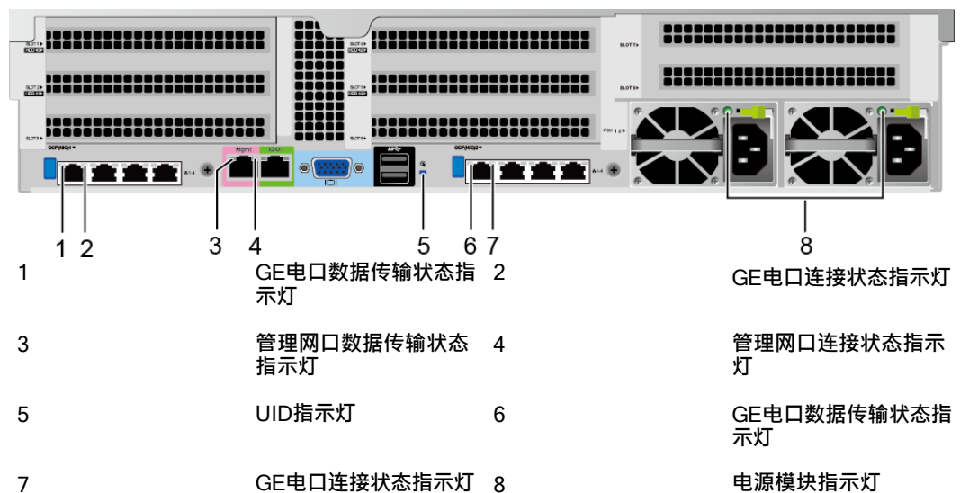
图 3-14 后面板指示灯
