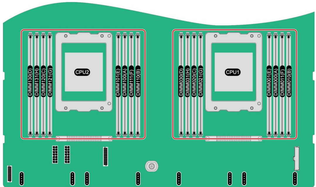
图 3-28 内存槽位编号
