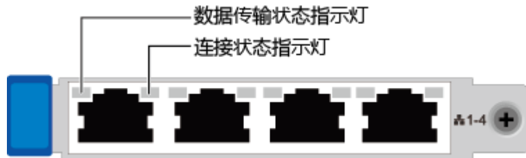
图 3-15 TM210 ( 4*GE 电口 )
