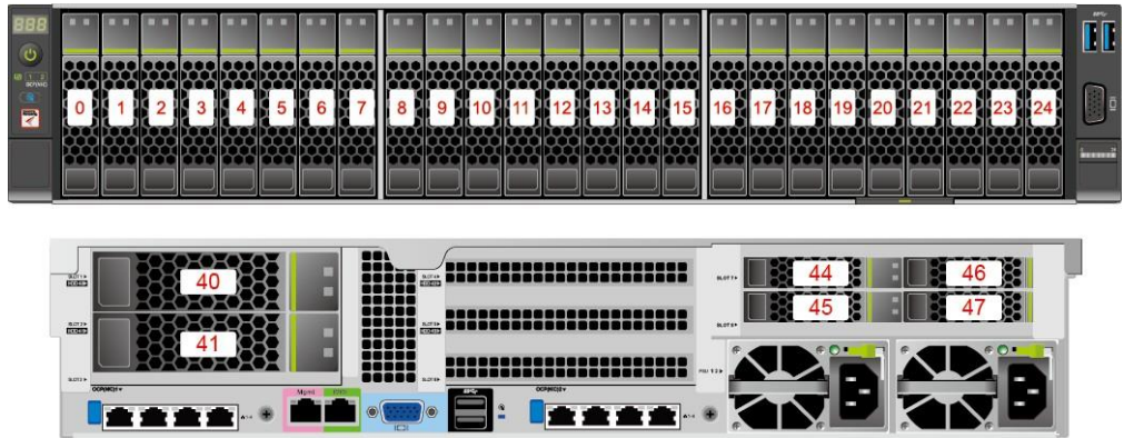
图 3-18 25x2.5 英寸硬盘 EXP 配置
