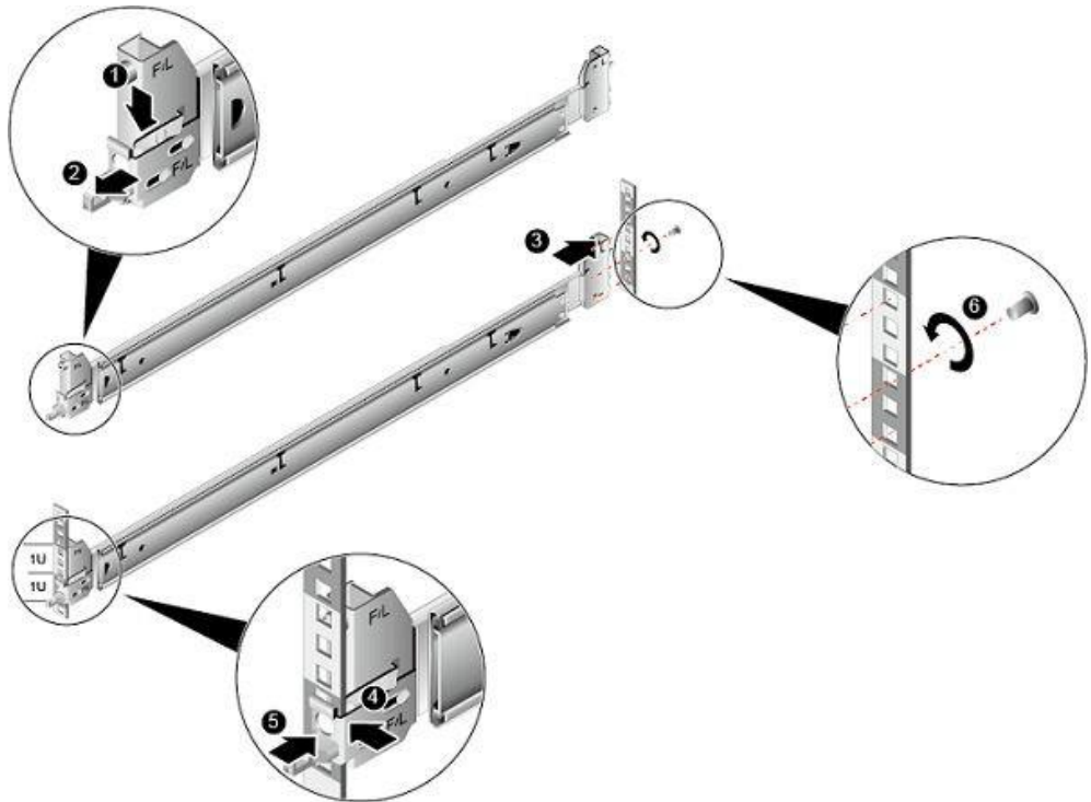
图 6-10 安装抱轨前后端
