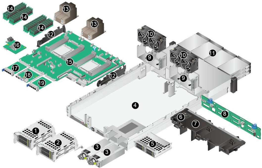
图 2-2 部件
