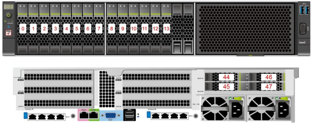
图 3-23 8x2.5 SAS/SATA+6x2.5 NVMe 硬盘配置硬盘编号
