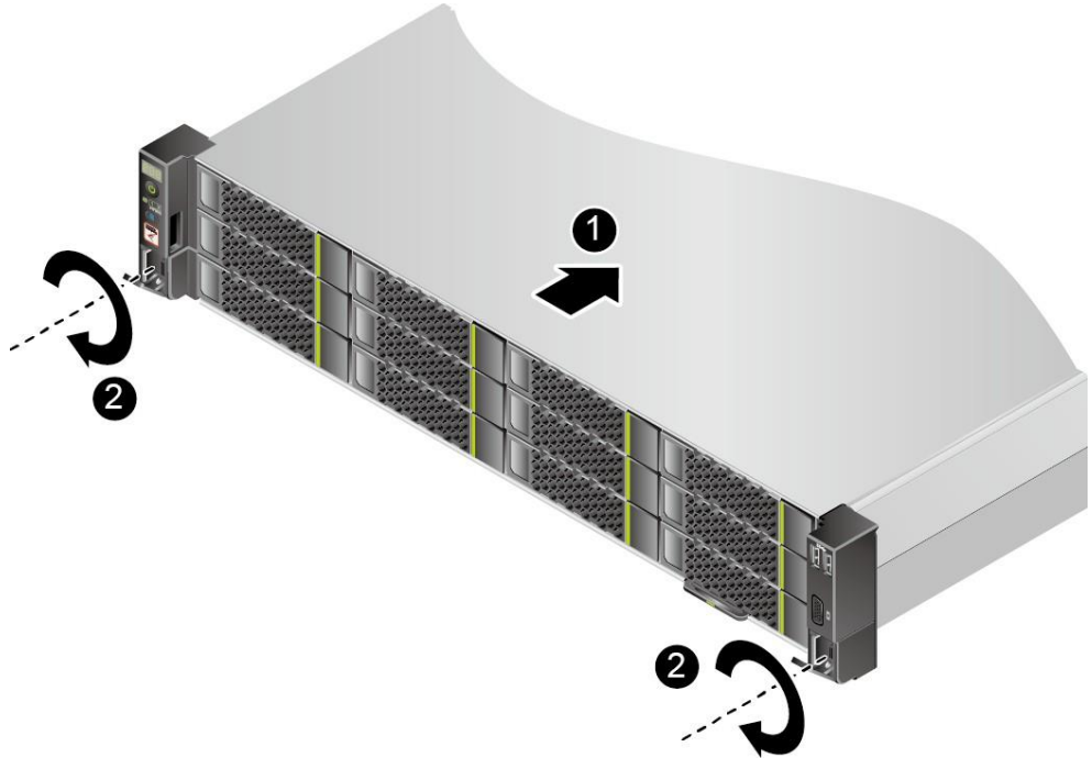
图 6-7 安装服务器
