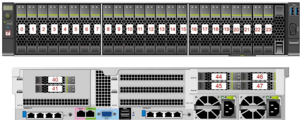
图 3-25 24x2.5 英寸硬盘 RAID 直通配置的硬盘编号
