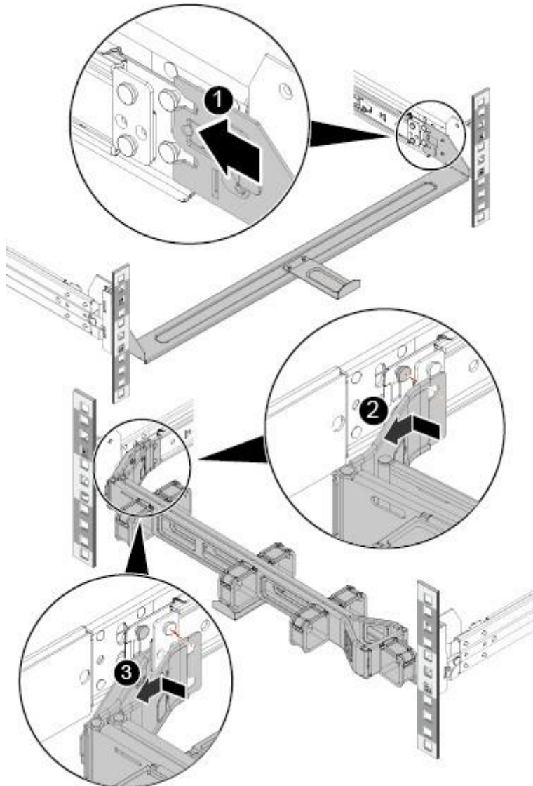
图 6-15 安装理线架
