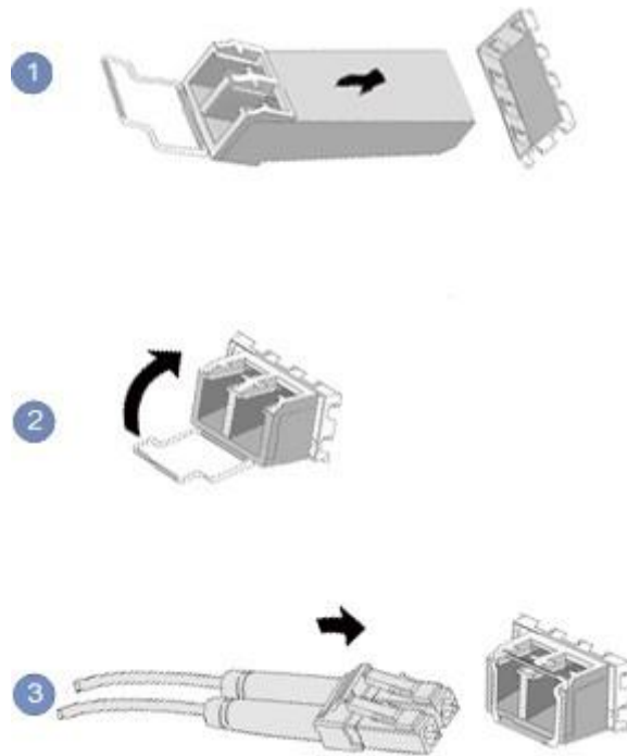
图 6-18 连接光纤
