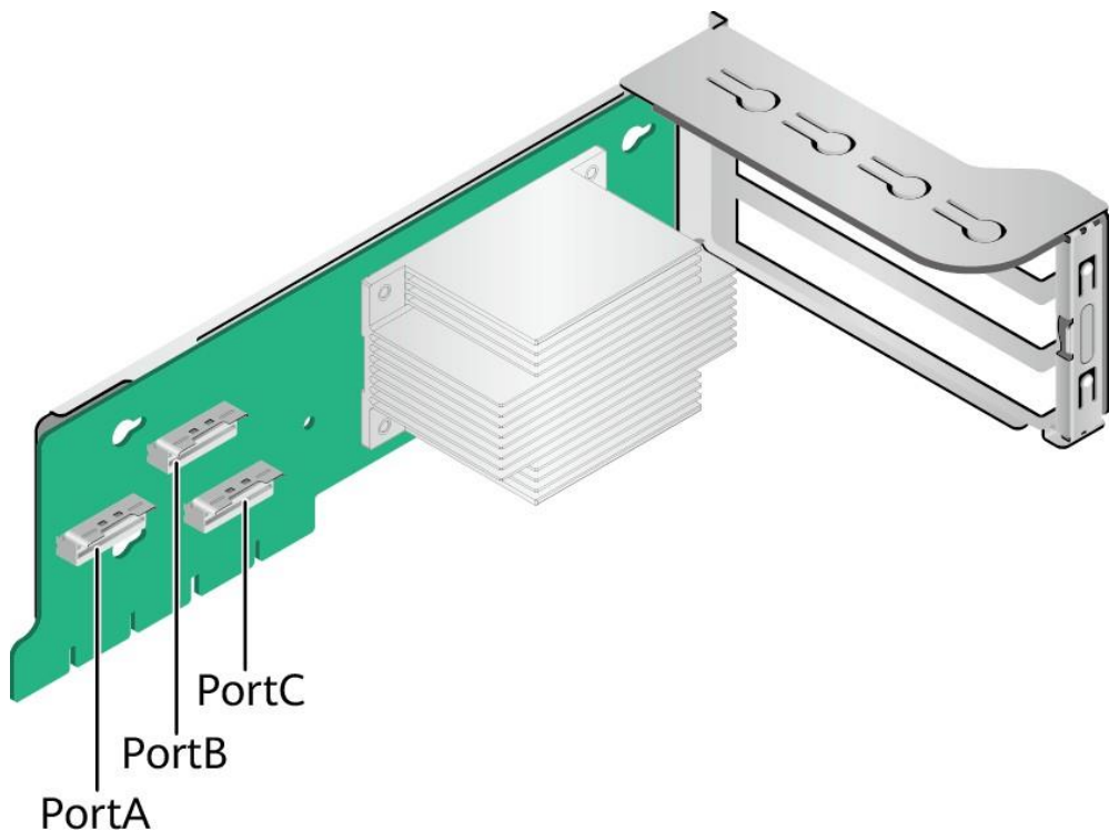
图 3-31 12NVMe 专用 Riser 卡 3
