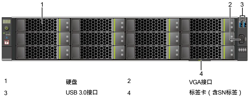
图 3-1 12x3.5 英寸硬盘配置的前面板组件
