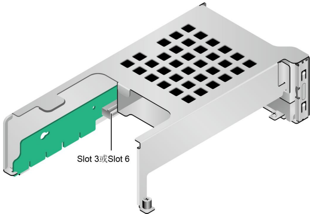
图 3-33 1x16 Riser 卡 4
