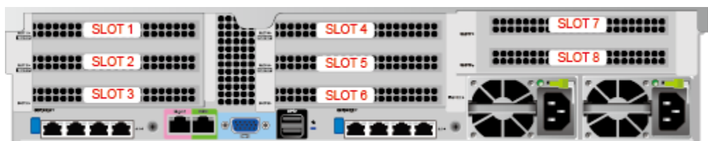
图 3-37 PCIe 插槽
