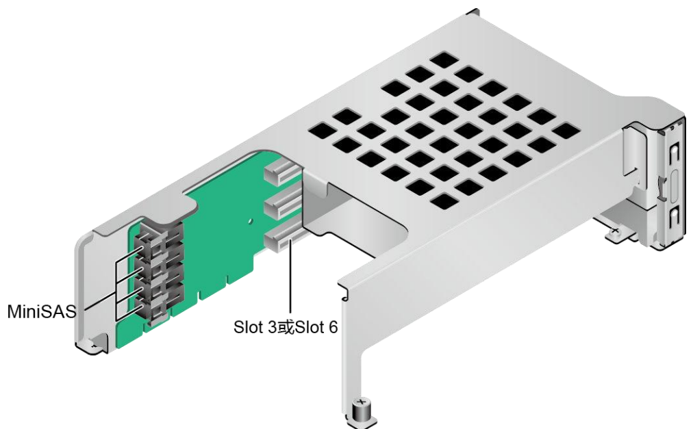
图 3-34 SAS Riser 卡 5
