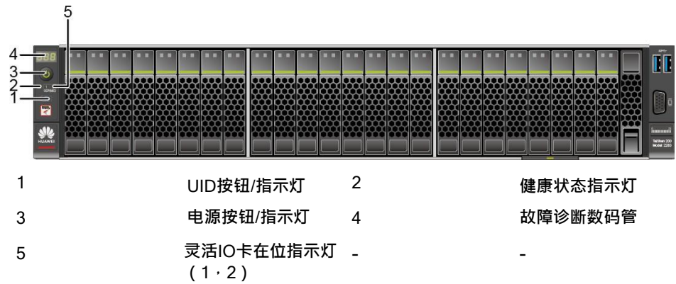
图 3-12 24x2.5 英寸硬盘配置前面板指示灯和按钮
