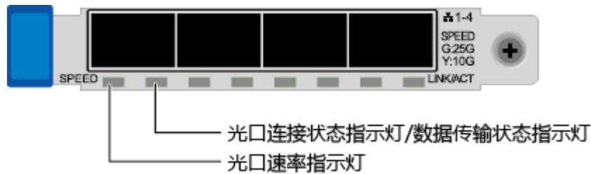
图 3-17 TM280 ( 4x25GE 光口 )
