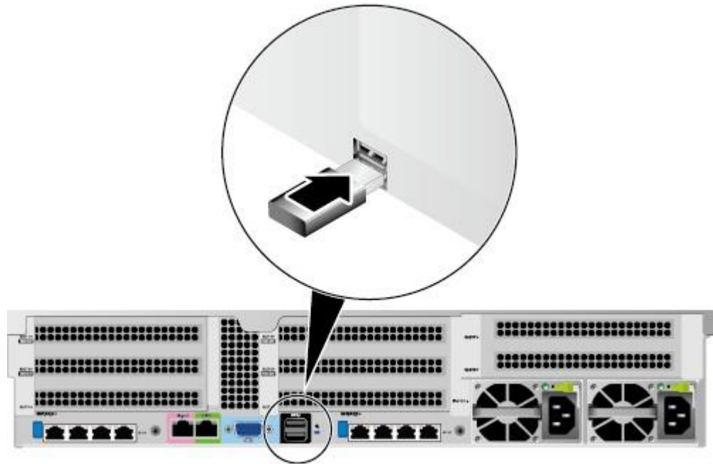
图 6-21 连接 USB 接口
