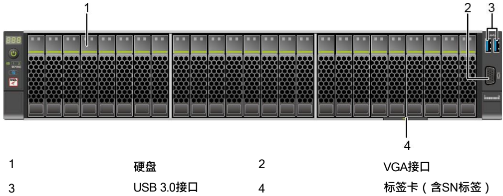
图 3-3 25x2.5 英寸硬盘配置的前面板组件
