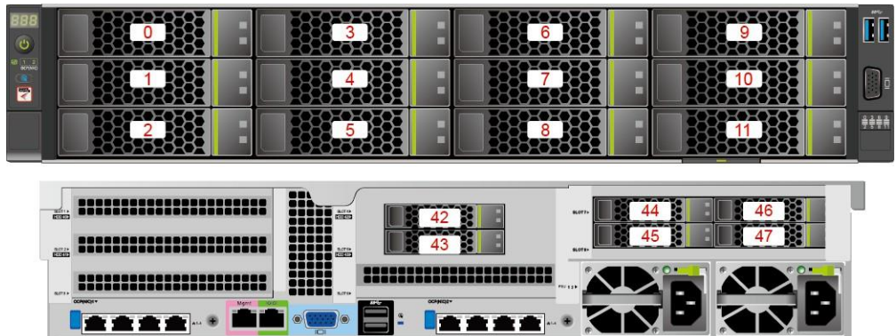
图 3-20 12x3.5 英寸硬盘直通配置
