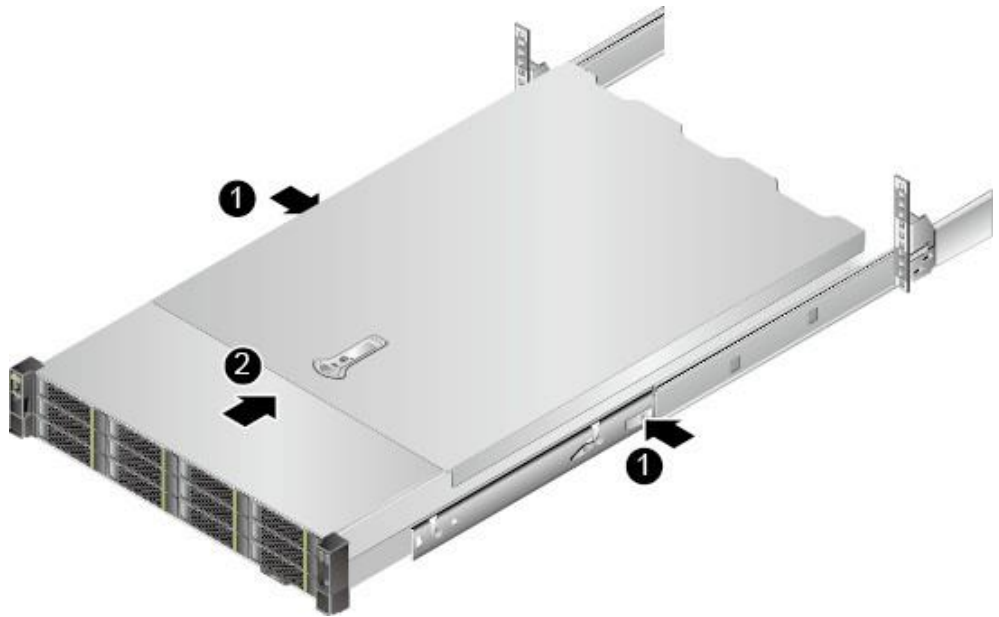
图 6-13 将服务器推入抱轨
