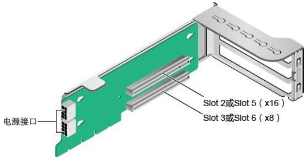
图 3-30 1x8+1x16 Riser 卡 2
