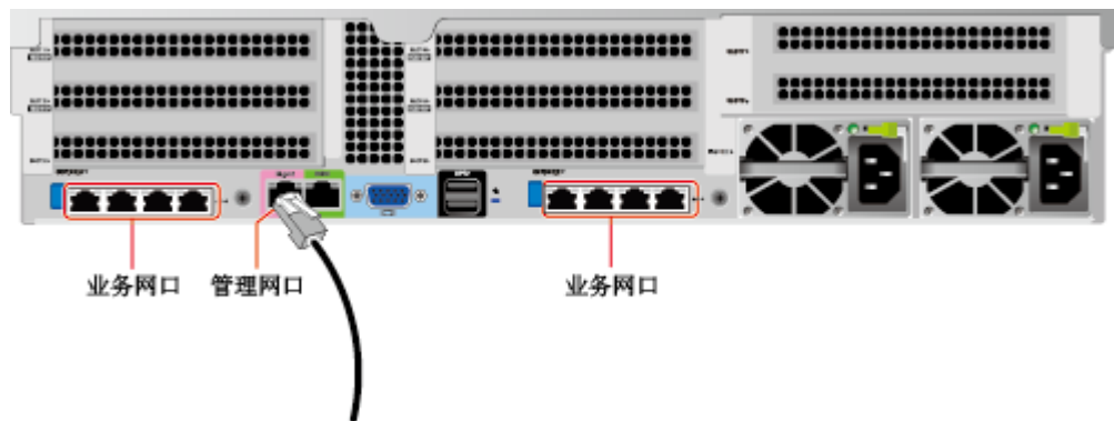
图 6-17 连接网线
