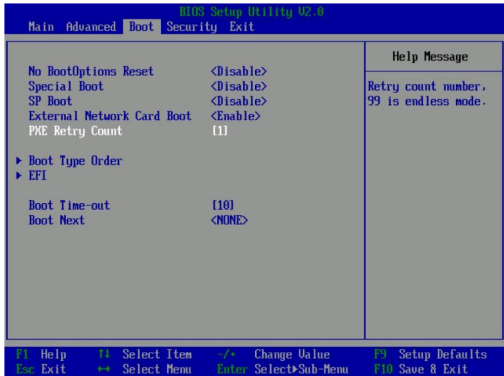
图 6-44 Boot 界面
