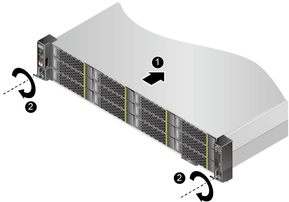
图 6-9 安装服务器
