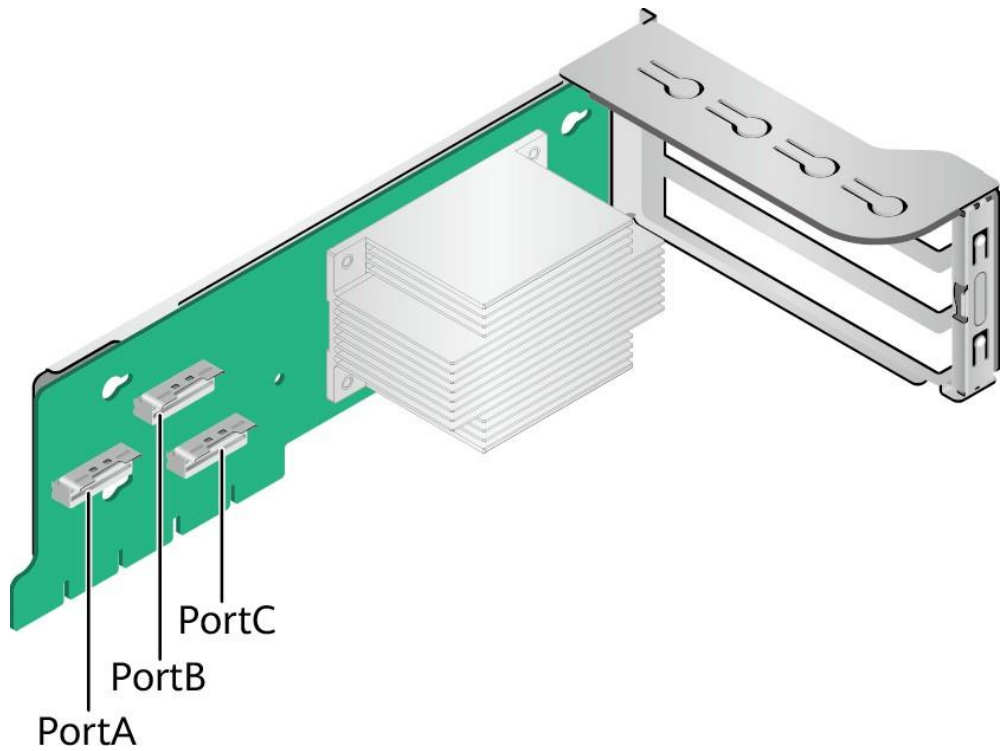
图 3-32 6NVMe 专用 Riser 卡 3
