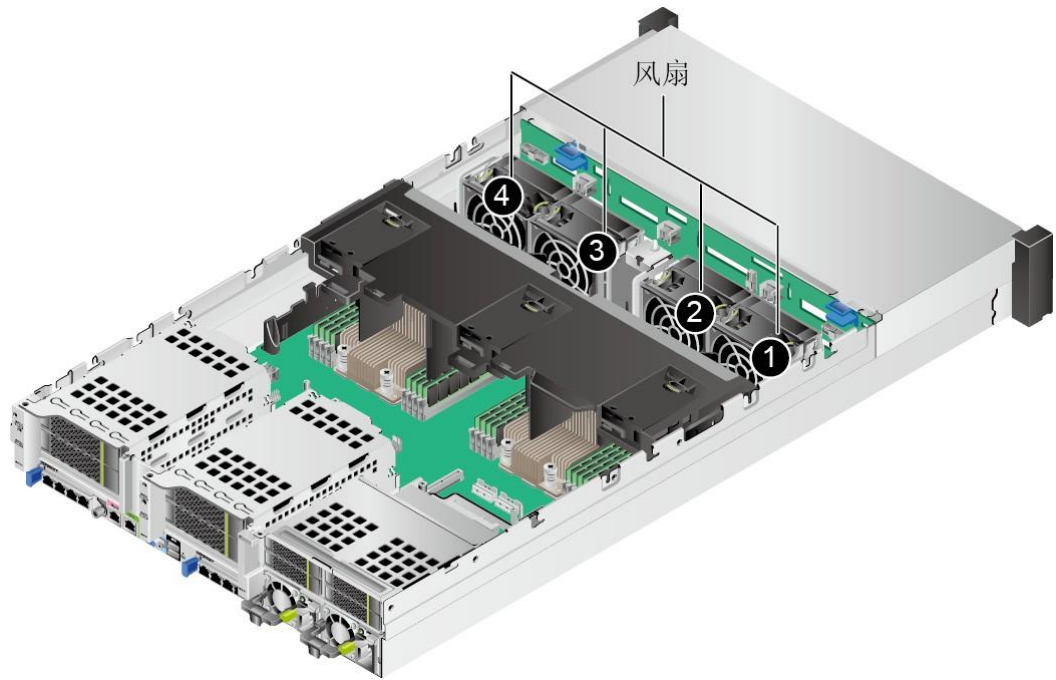
图 3-38 风扇位置图
