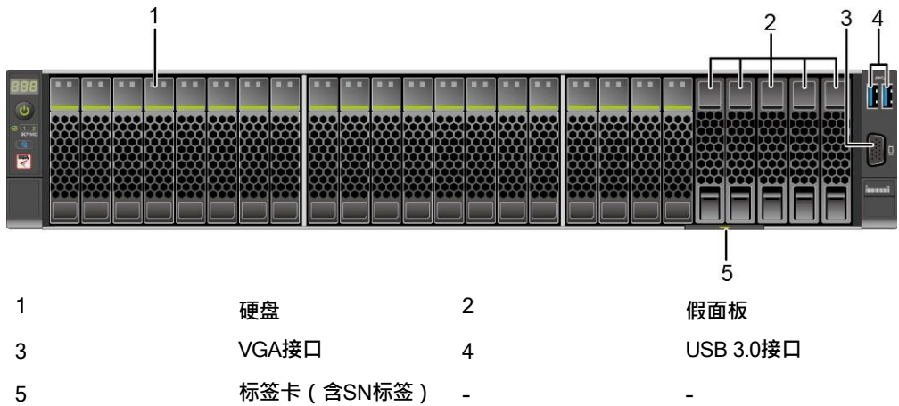
图 3-4 8x2.5 SAS/SATA+12x2.5 NVMe 硬盘配置的前面板组件
