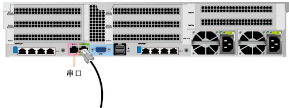
图 6-22 连接串口线缆
