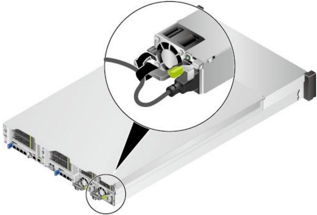
图 6-24 固定电源线缆
