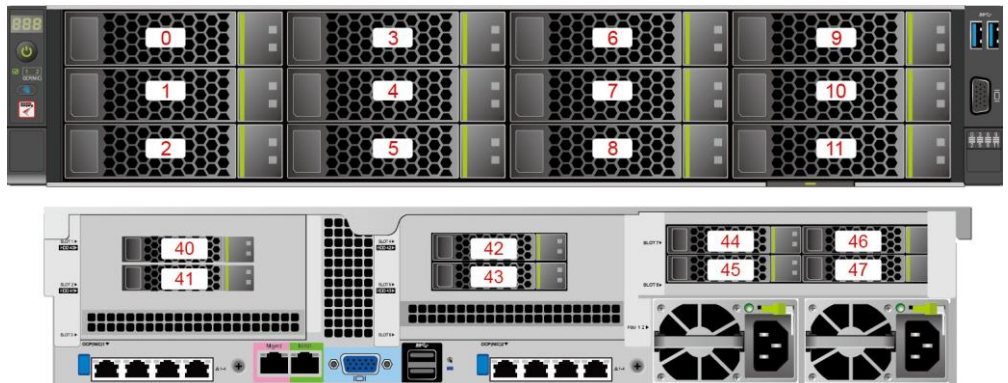
图 3-21 12x3.5 英寸硬盘 RAID 直通配置
