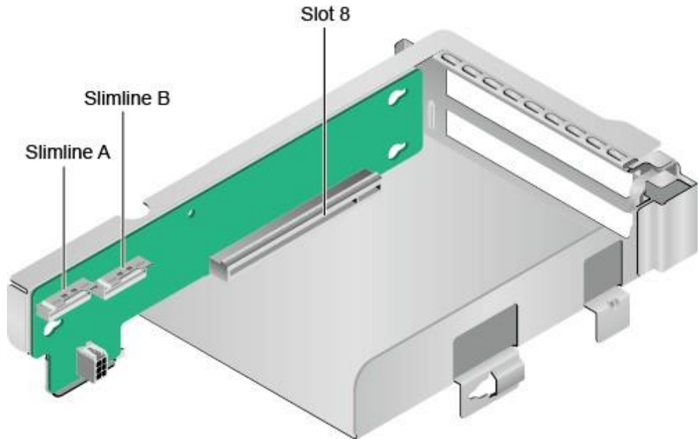
图 3-36 1x16 Riser 卡 7
