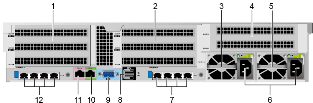
图 3-13 后面板组件
